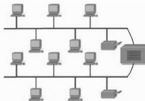
Domínio de Colisão estendido pelo Repetidor
