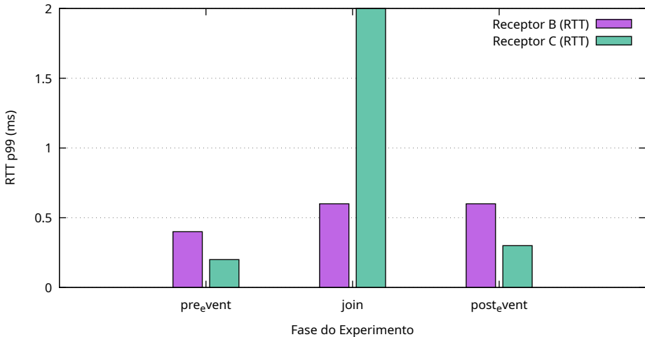
Desempenho por Fase - Cenário S2 (Impacto do Join Multicast)
