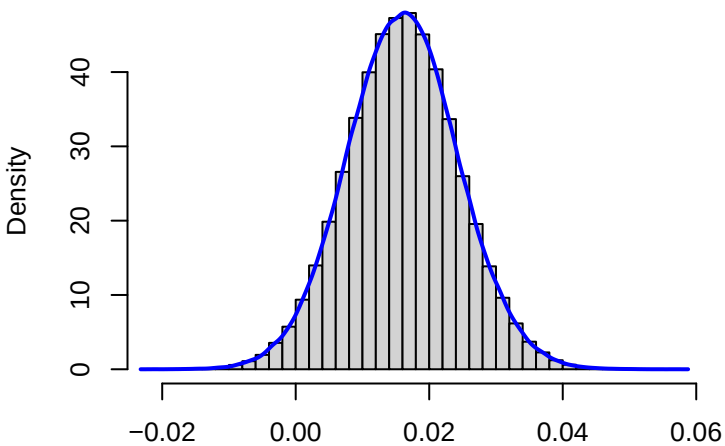
Posterior of \theta_{1200,2}
