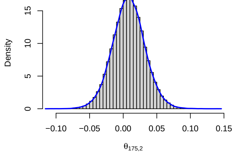
Posterior of \theta_{175,2}
