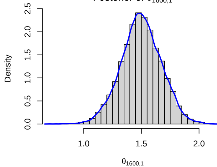
Posterior of \theta_{1600,1}
