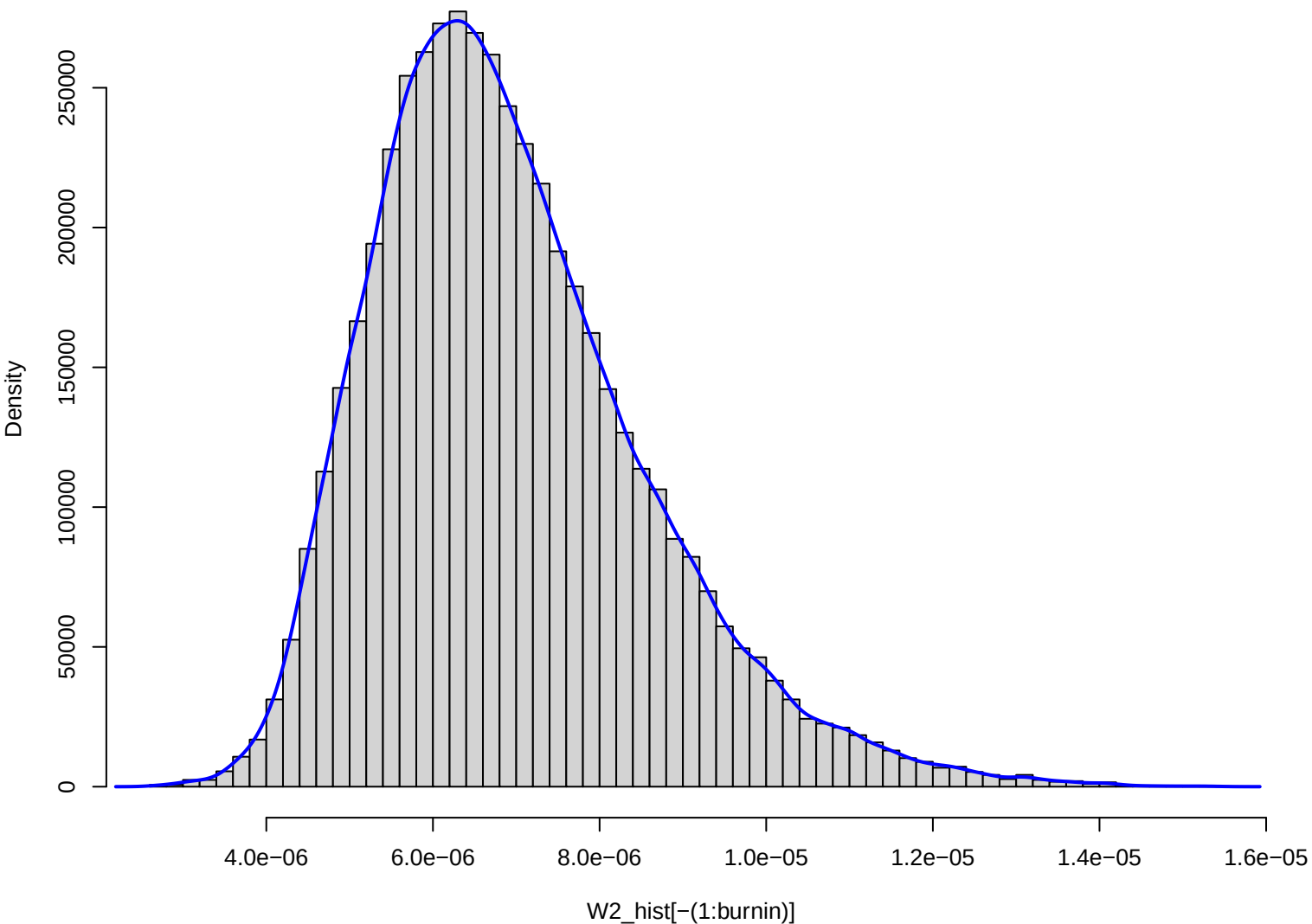
Posterior of W2
