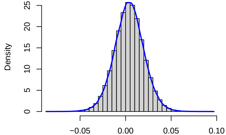
Posterior of \theta_{100,2}
