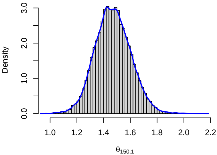
Posterior of \theta_{150,1}
