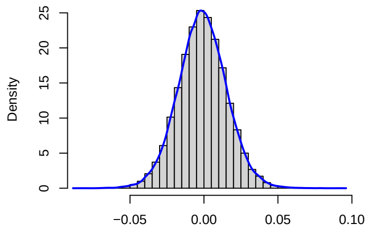
Posterior of \theta_{175,2}
