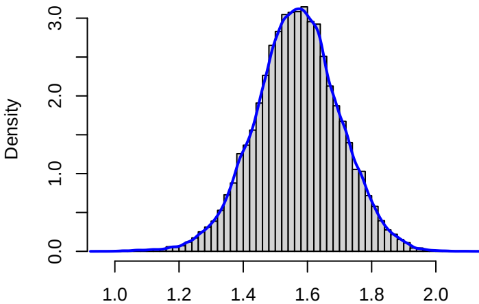
Posterior of \theta_{50,1}
