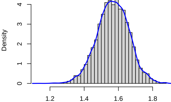
Posterior of \theta_{400,1}
