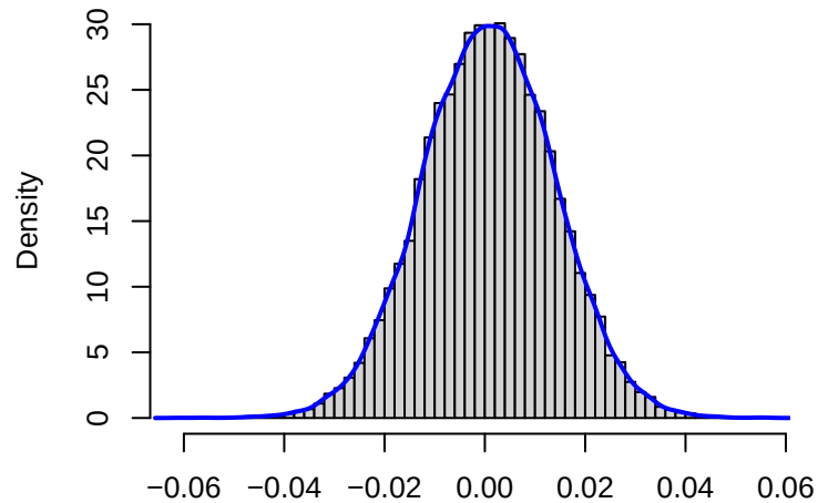
Posterior of \theta_{1600,2}
