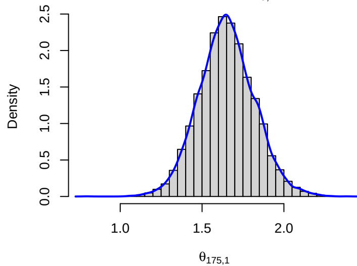
Posterior of \theta_{175,1}
