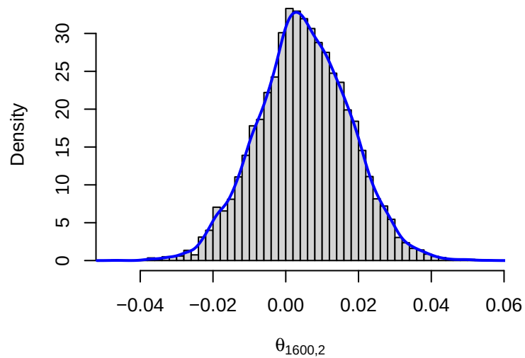
Posterior of \theta_{1600,2}
