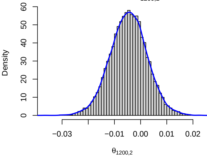
Posterior of \theta_{1200,2}
