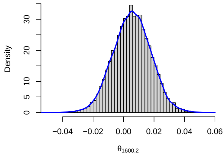
Posterior of \theta_{1600,2}
