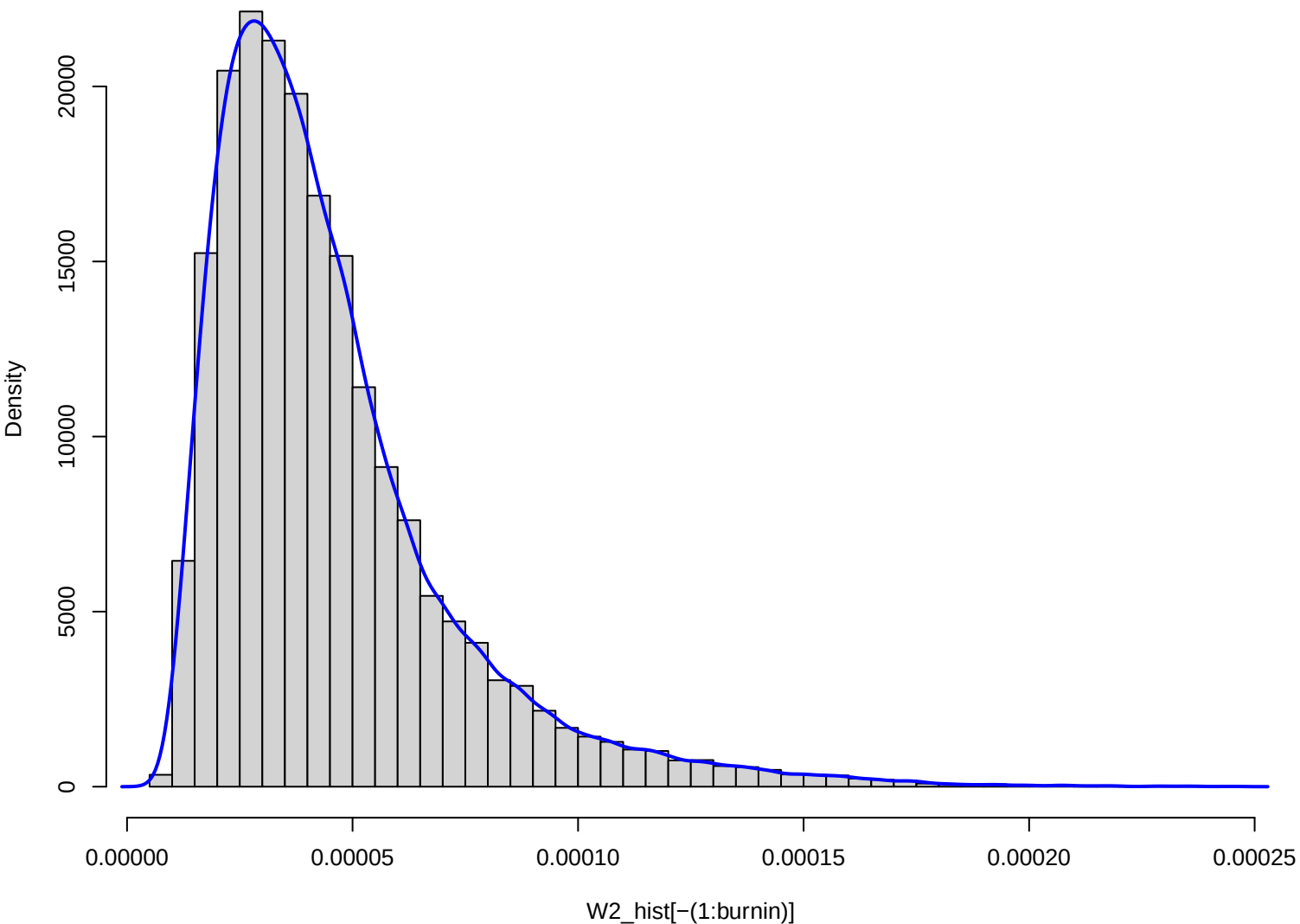
Posterior of W2
