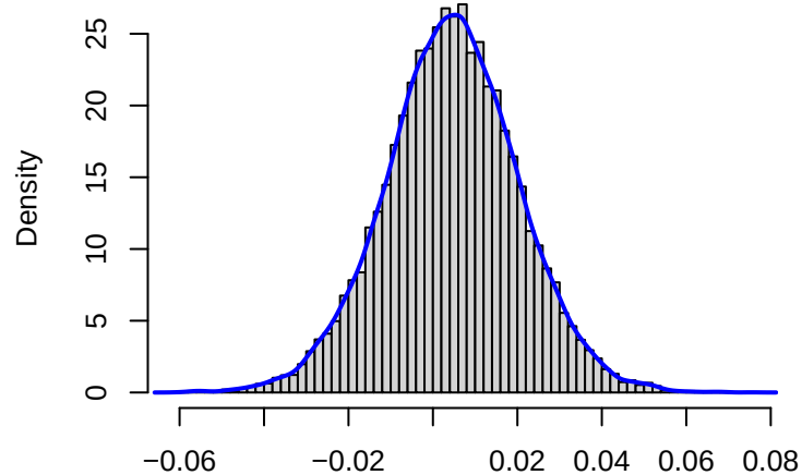
Posterior of \theta_{100,2}
