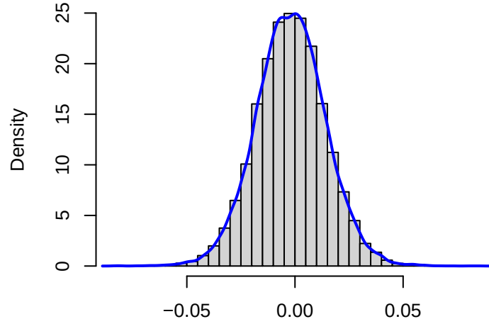
Posterior of \theta_{175,2}
