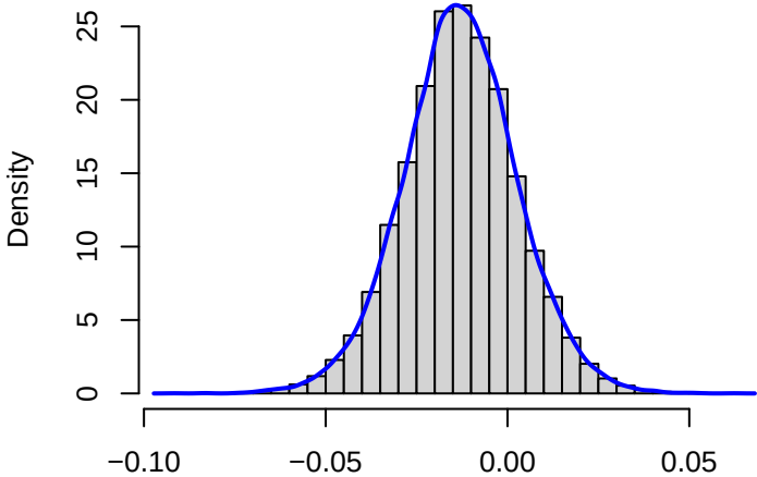
Posterior of \theta_{50,2}
