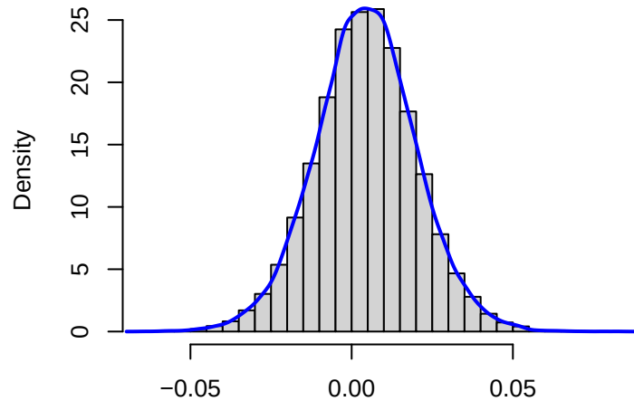
Posterior of \theta_{100,2}
