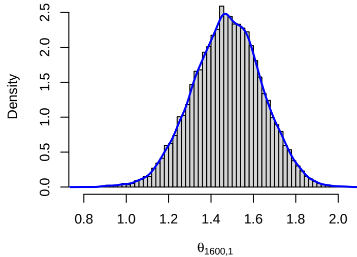
Posterior of \theta_{1600,1}
