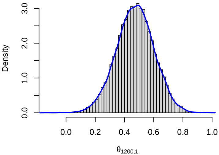
Posterior of \theta_{1200,1}
