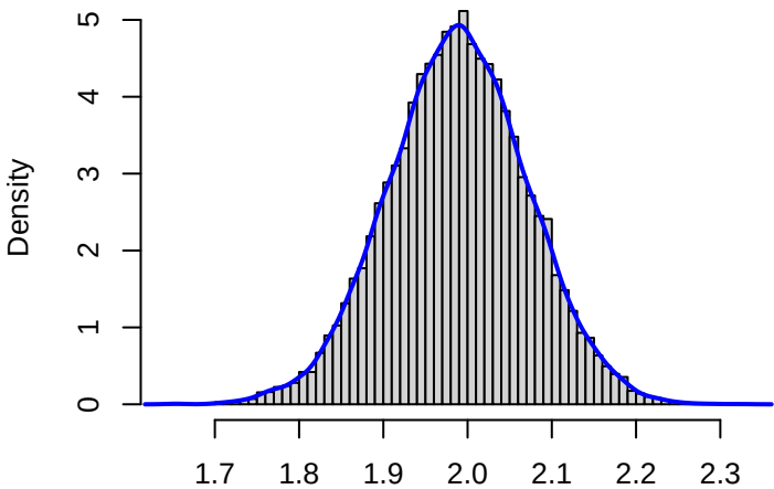
Posterior of \theta_{400,1}
