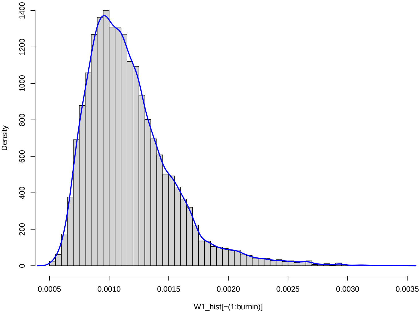
Posterior of W1
