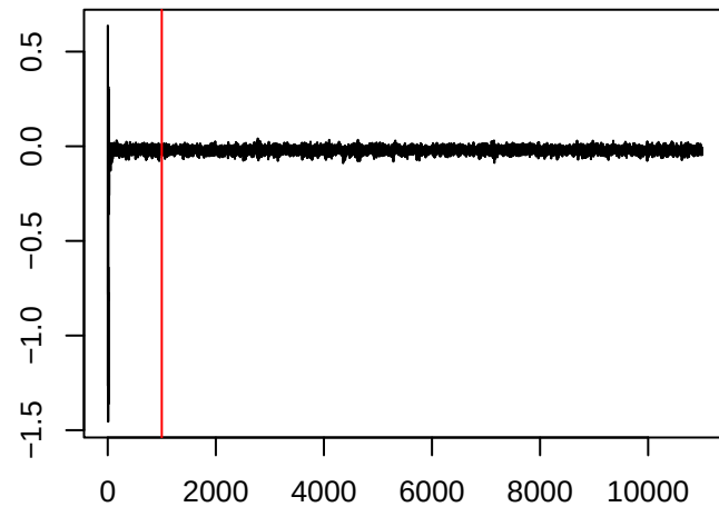
\theta_{100,2}
