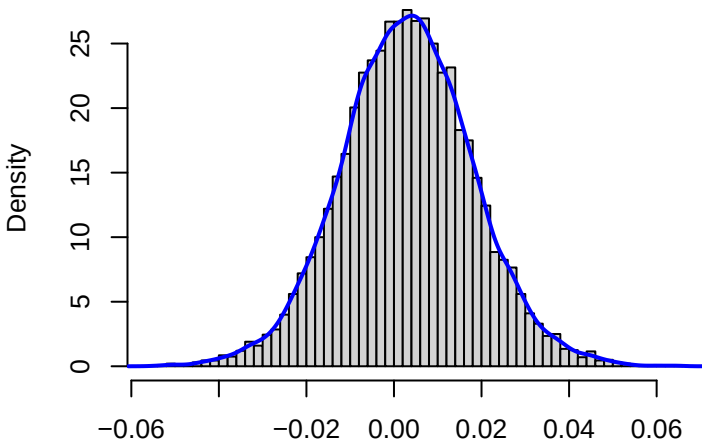
Posterior of \theta_{150,2}
