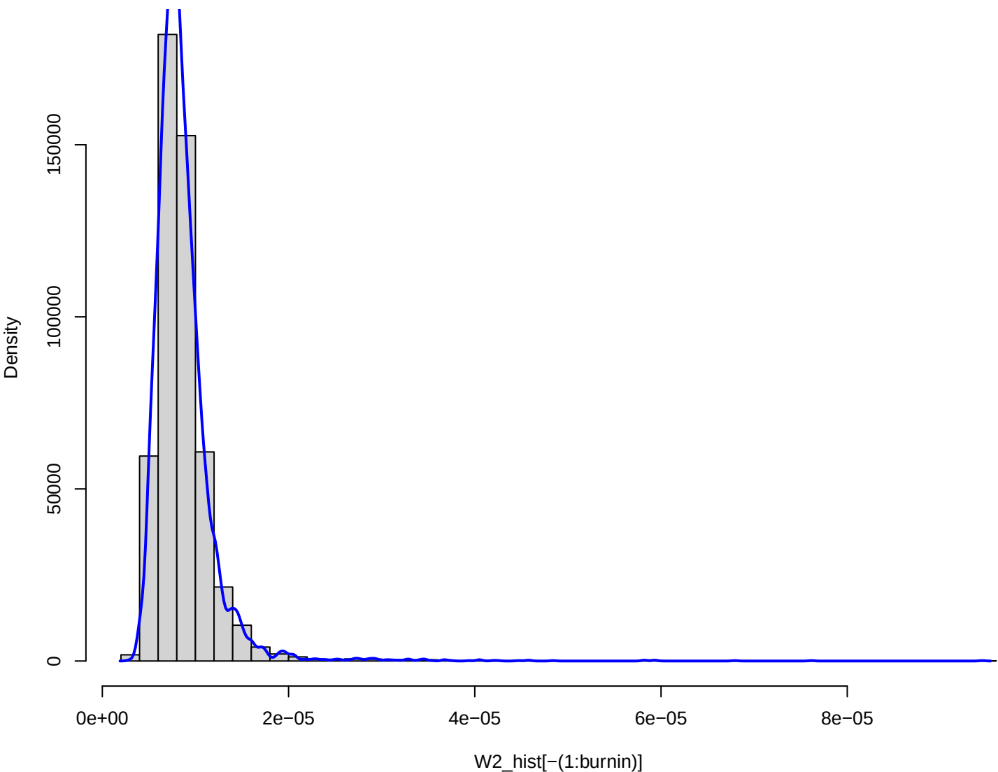
Posterior of W2
