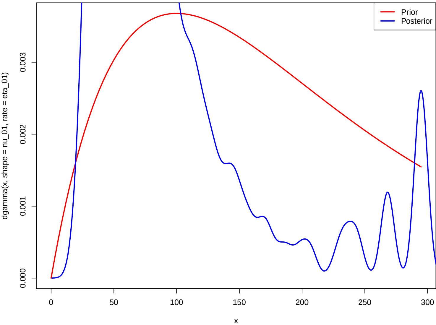
phi1 prior vs. posterior
