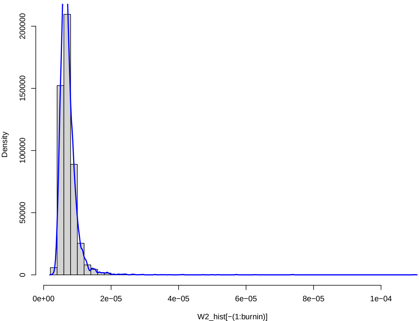
Posterior of W2
