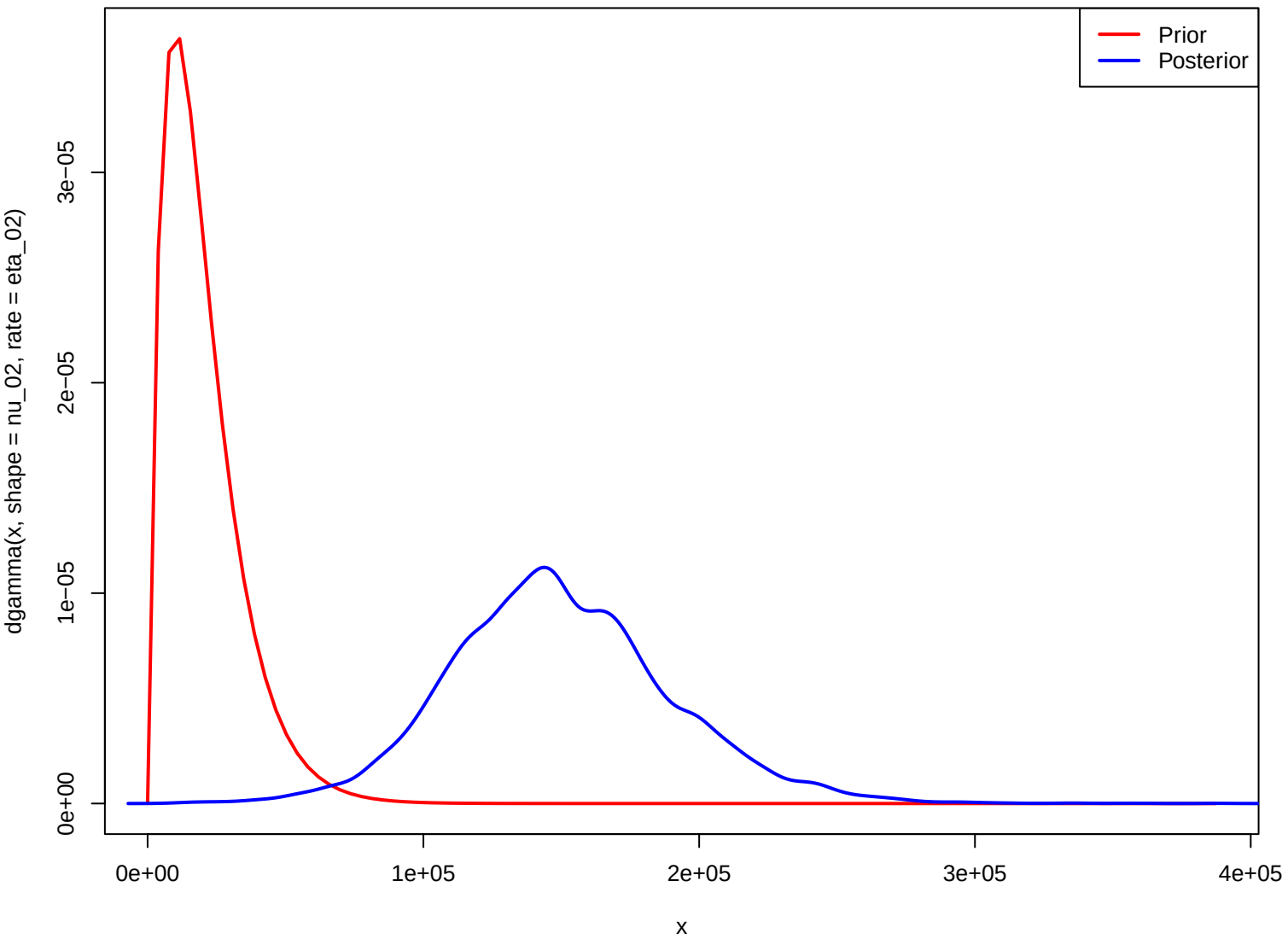
phi2 prior vs. posterior
