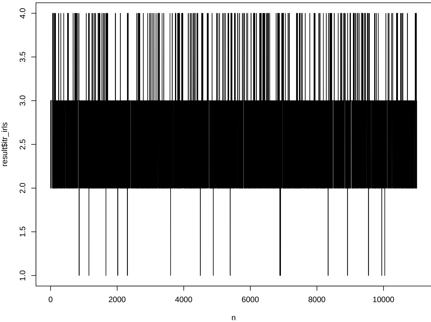
IRLS iterations per Gibbs step
