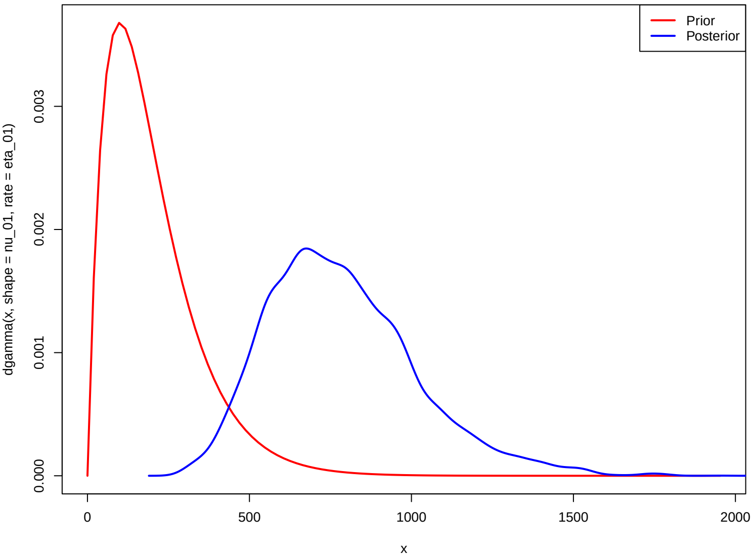
phi1 prior vs. posterior
