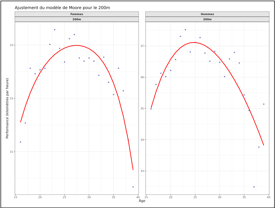
Figure 12: Ajustement du modèle de Moore sur le 200m. Points : meilleure performance annuelle par âge (km/h). Ligne rouge : courbe ajustée.
