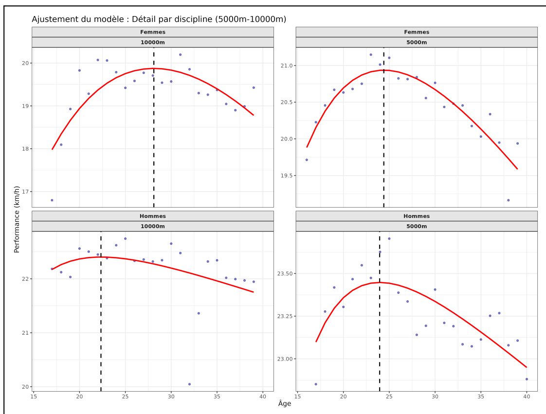
FIGURE 24 : Modèles de Moore pour les disciplines de fond
