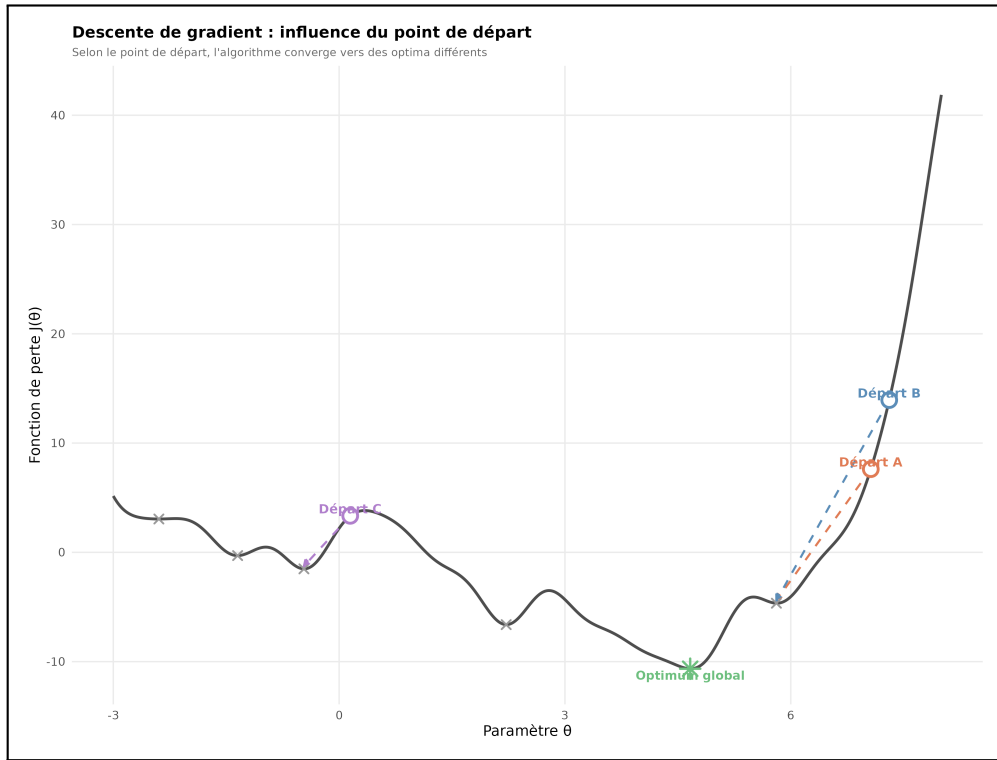
FIGURE 8 : Optimum local et descente de gradient
