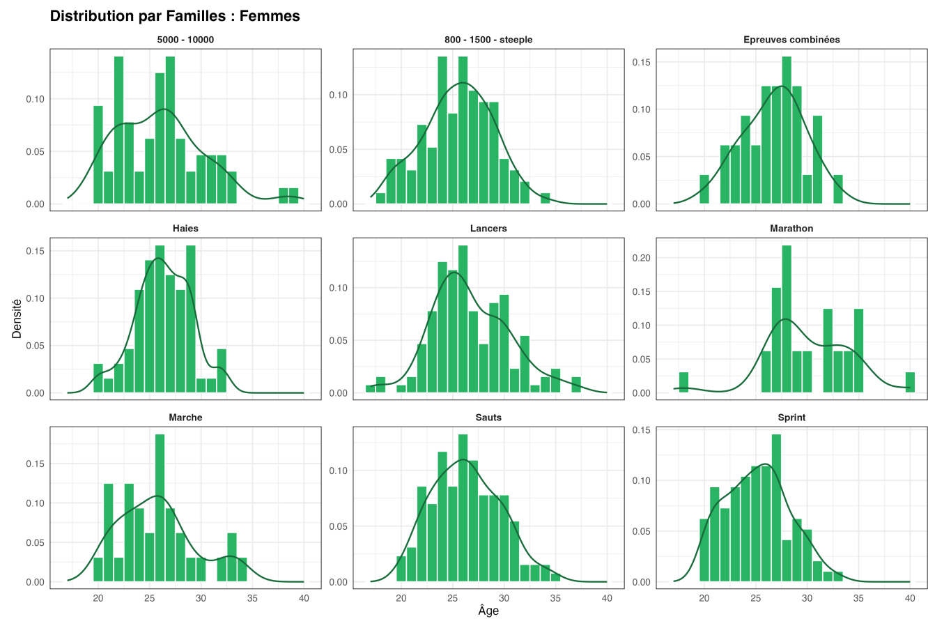
FIGURE 14 : Distributions par famille (femmes)
