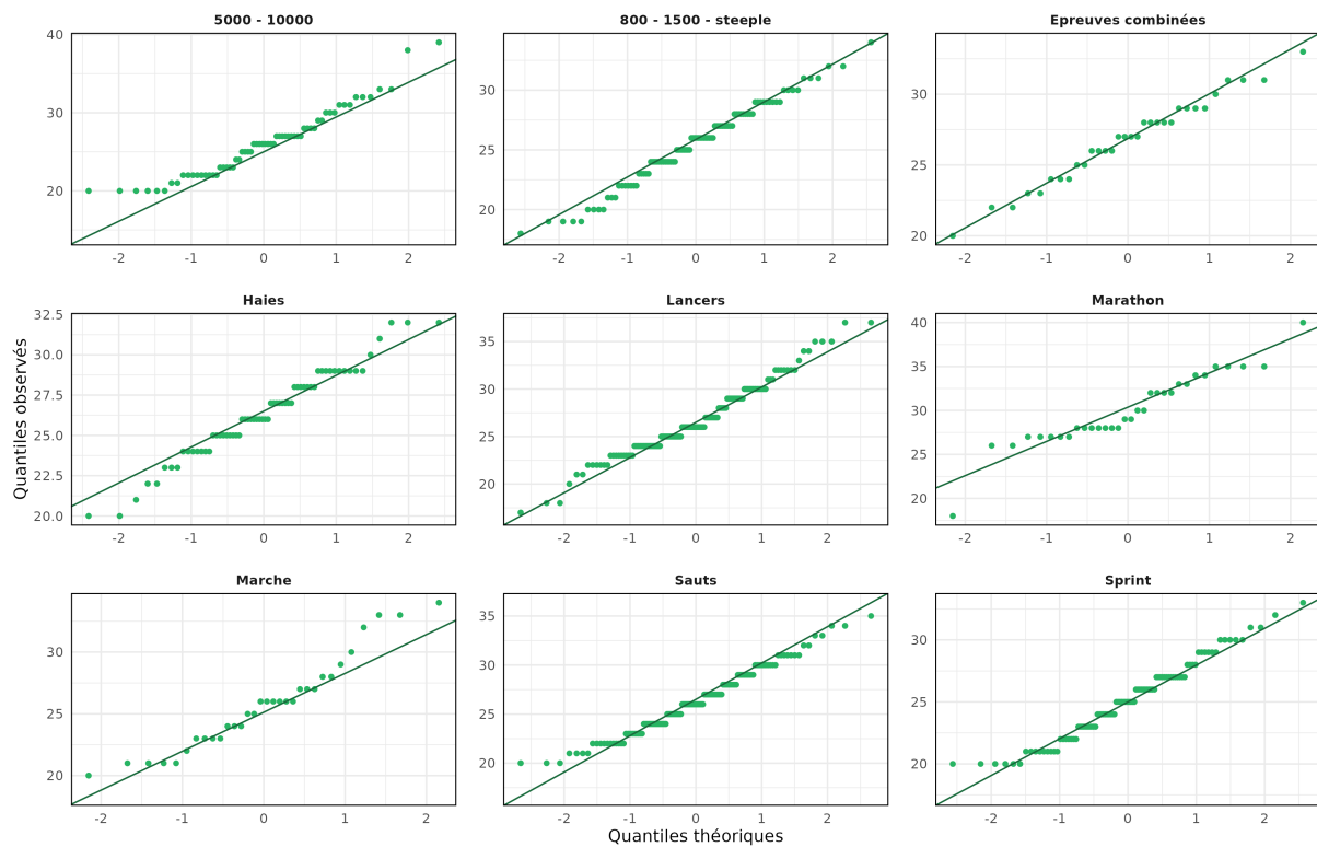
FIGURE 14 : QQ-plot de l'âge au pic (Femmes)
