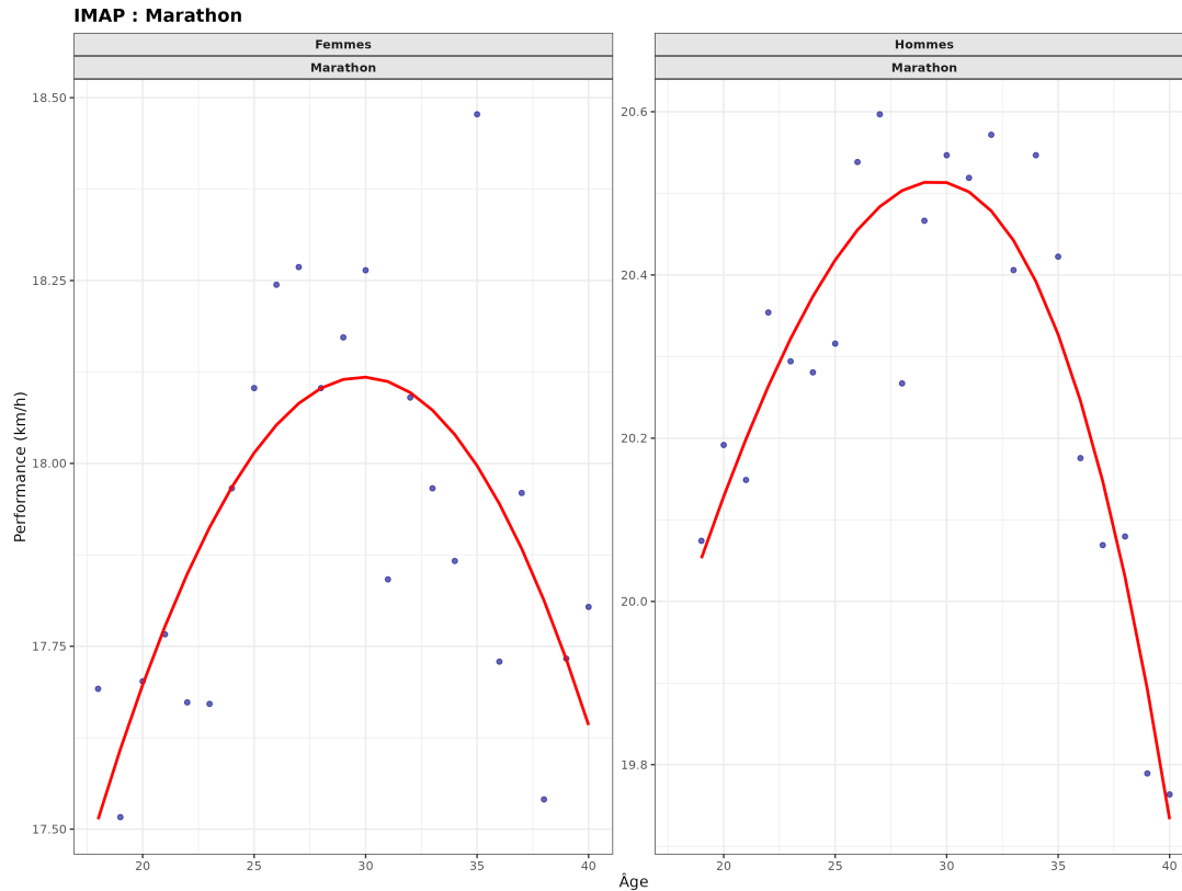
FIGURE 11 : Ajustement du modèle IMAP sur le marathon (hommes et femmes). Points : meilleure performance annuelle par âge. Ligne rouge : courbe ajustée.
