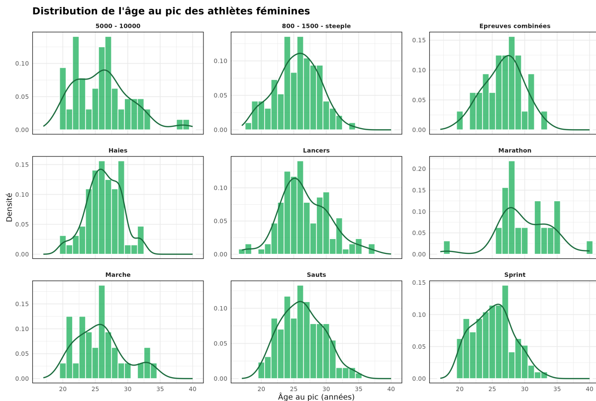
FIGURE 12 : Distributions de l'âge au pic de performance (Athlètes féminines)
