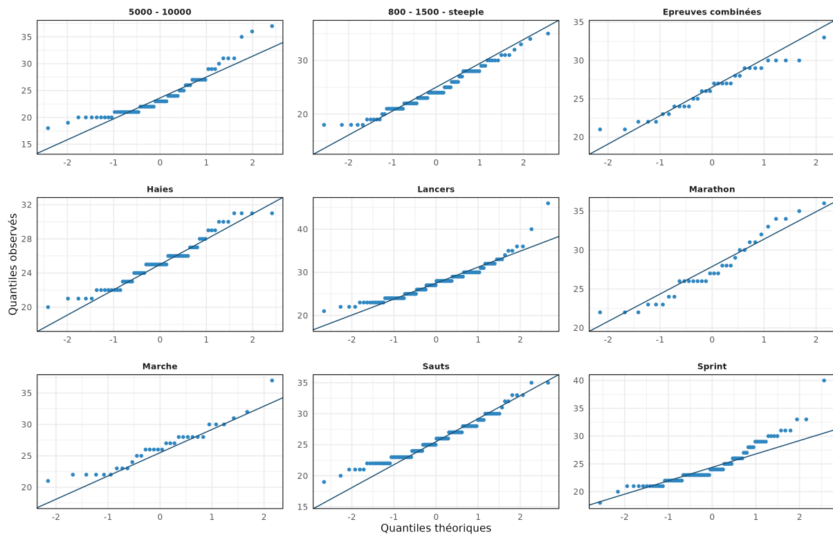
FIGURE 13 : QQ-plot de l'âge au pic (Hommes)
