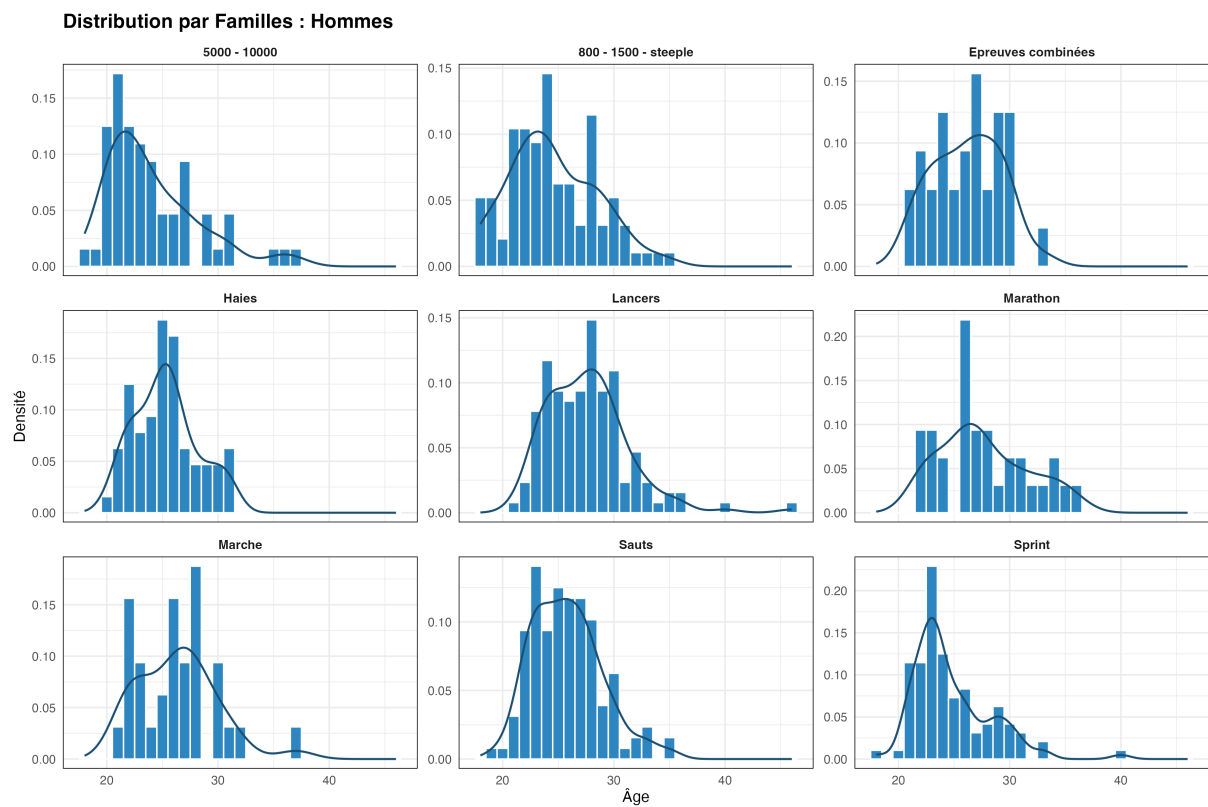
Figure 16: Distributions de l'âge au pic par famille (Hommes)
