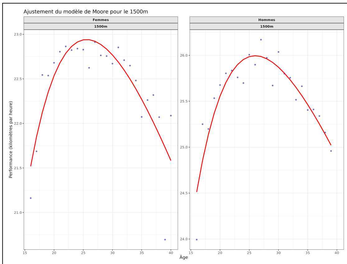
Figure 11: Ajustement du modèle de Moore sur le 1500m. Points : meilleure performance annuelle par âge (km/h). Ligne rouge : courbe ajustée.
