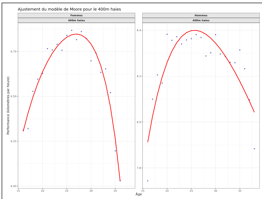
Figure 13: Ajustement du modèle de Moore sur le 400m haies. Points : meilleure performance annuelle par âge (km/h). Ligne rouge : courbe ajustée.
