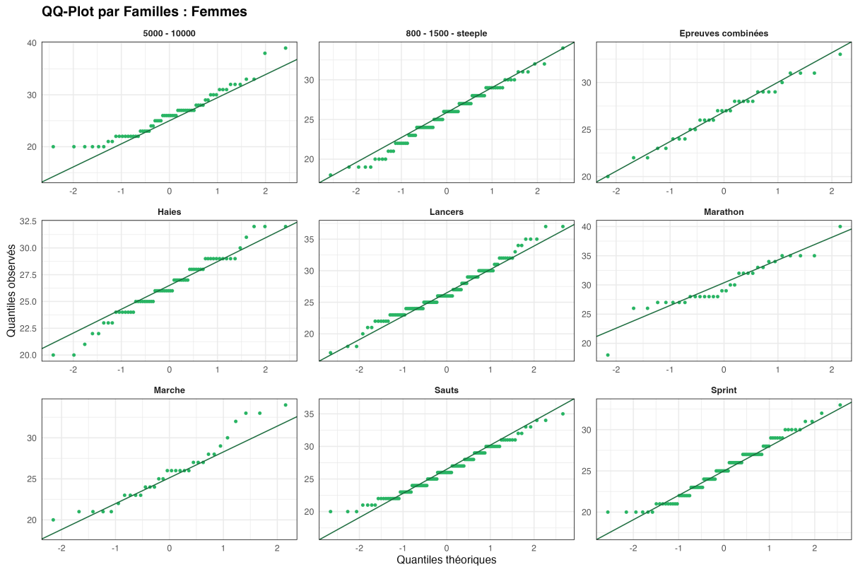
Figure 21: QQ-plots par famille (Femmes)
