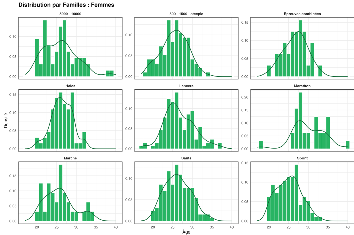
Figure 17: Distributions de l'âge au pic par famille (Femmes)
