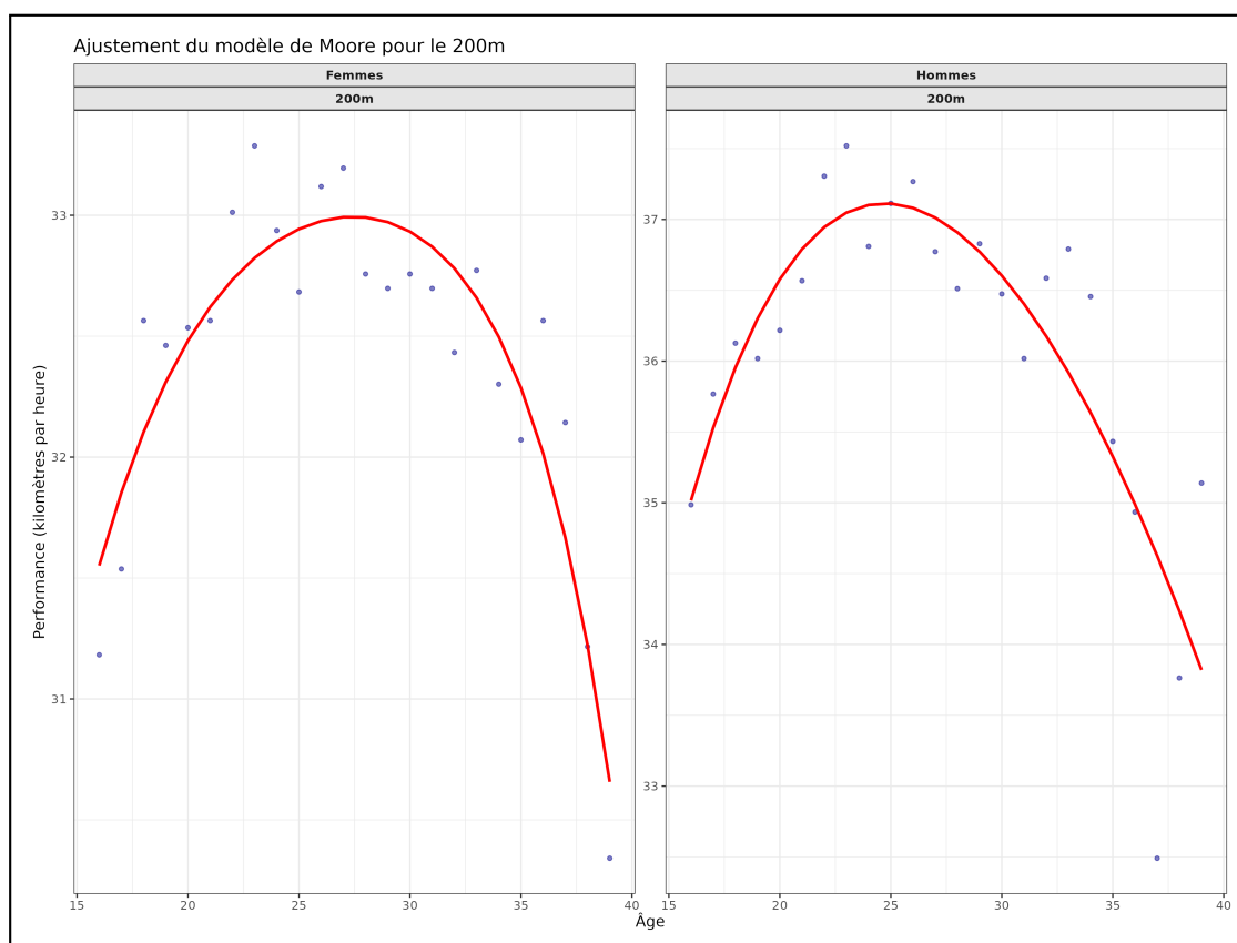
Figure 12: Ajustement du modèle de Moore sur le 200m. Points : meilleure performance annuelle par âge (km/h). Ligne rouge : courbe ajustée.
