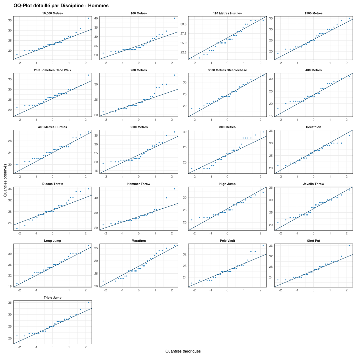
Figure 18: QQ-plots par discipline (Hommes)
