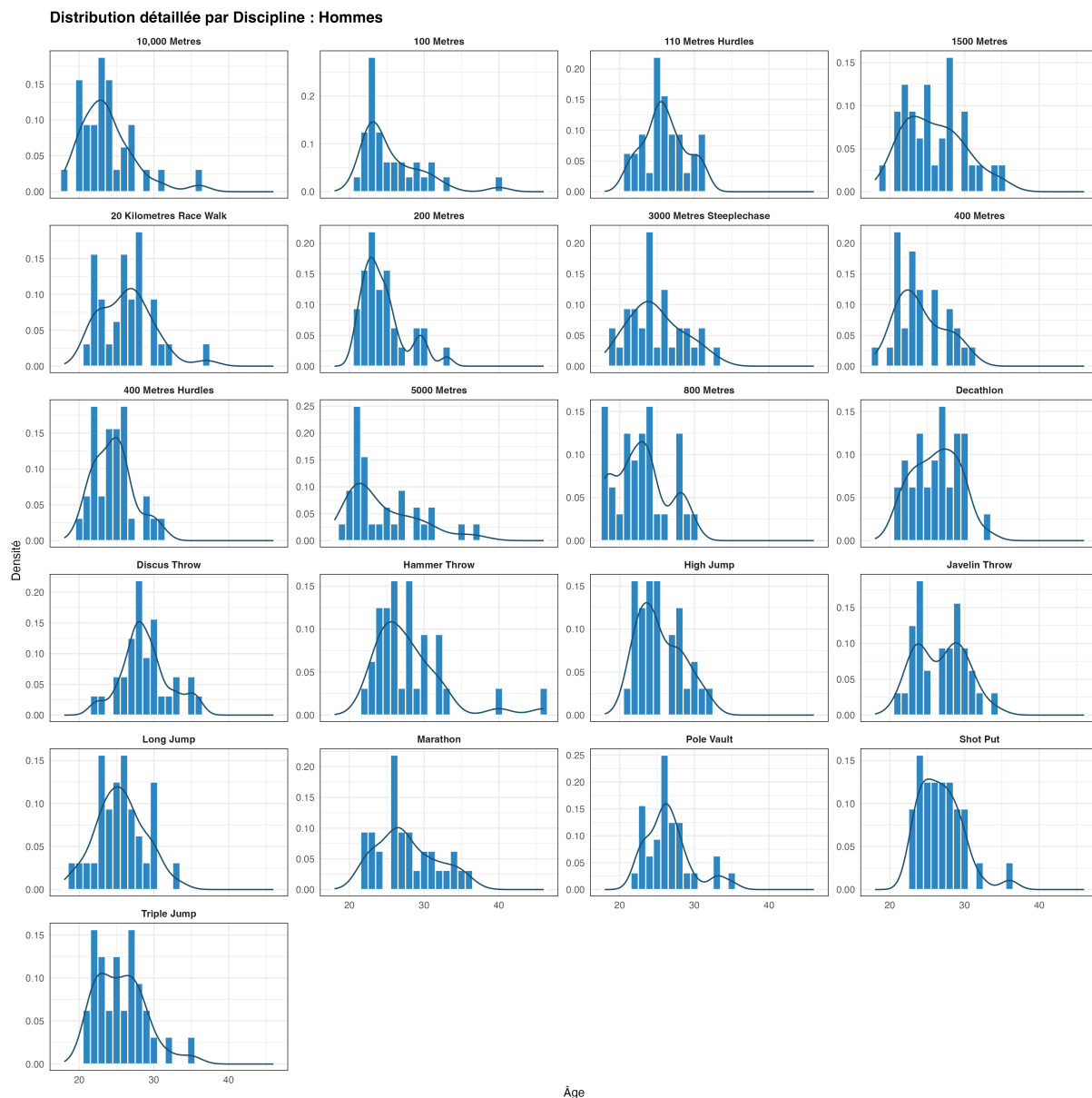
Figure 14: Distributions de l'âge au pic par discipline (Hommes)
