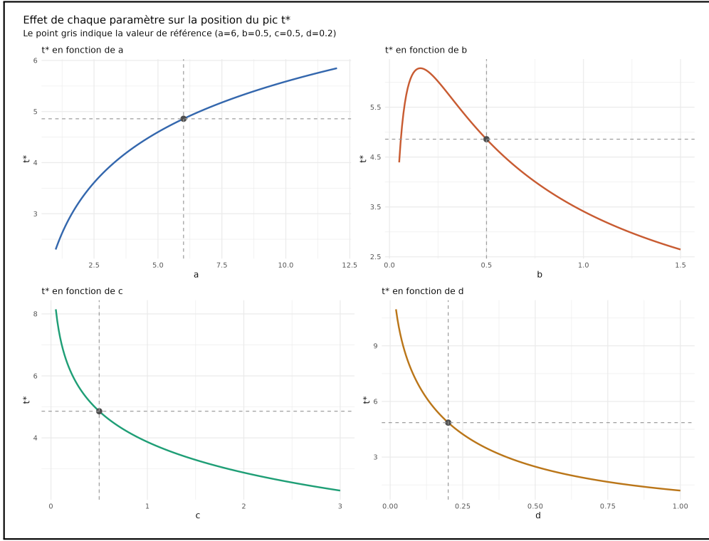
Figure 6: Effet des paramètres sur l'âge au pic théorique ( t_{pic} )
