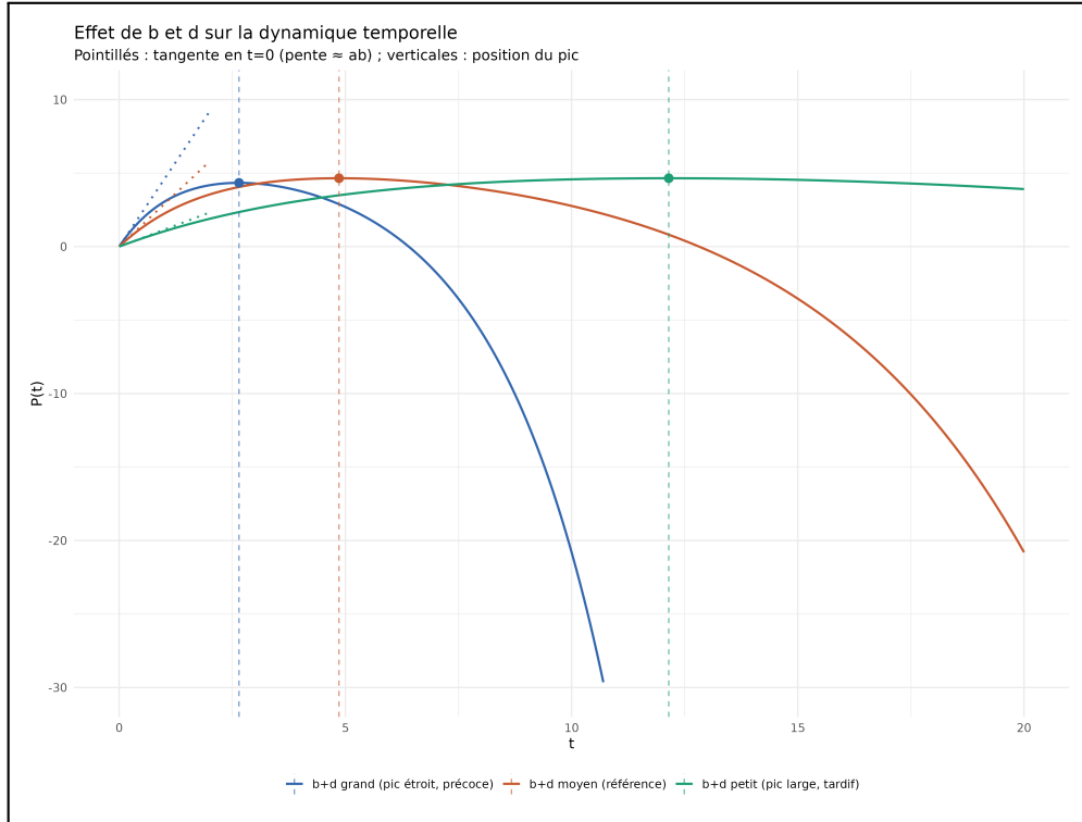
Figure 5: Effet des paramètres b et d sur la modélisation
