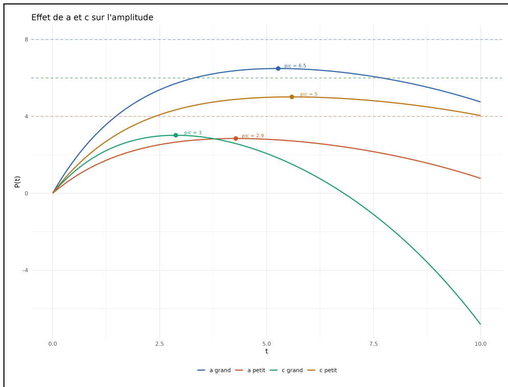
Figure 4: Effet des paramètres a et c sur la modélisation
