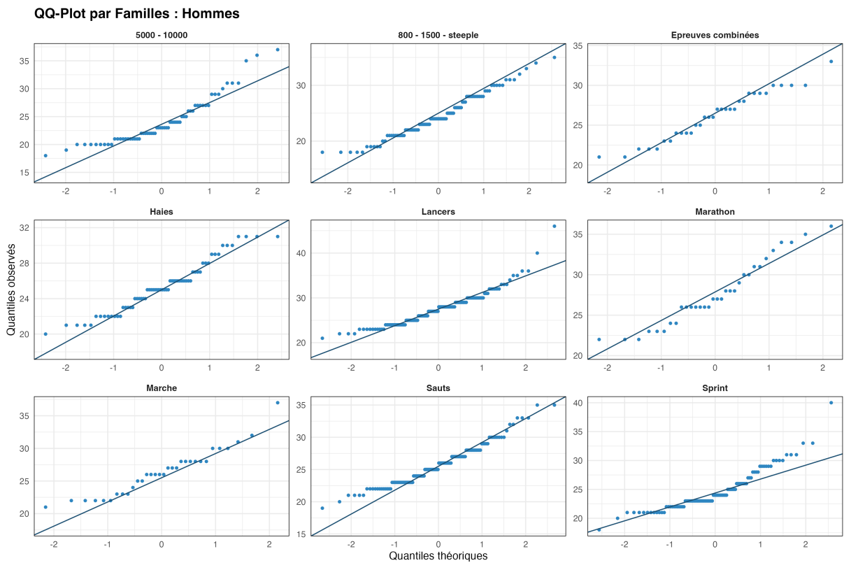
Figure 20: QQ-plots par famille (Hommes)
