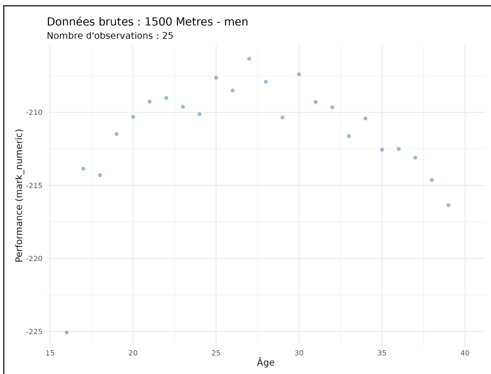
Figure 8: Meilleures performances par âge (1500 m - Hommes)
