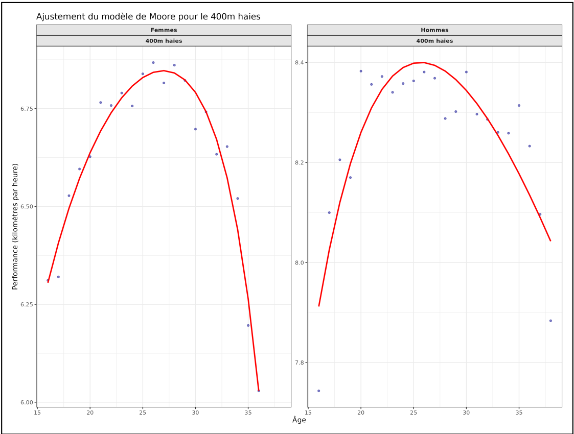
FIGURE 13 : Ajustement du modèle de Moore sur le 400m haies. Points : meilleure performance annuelle par âge (km/h). Ligne rouge : courbe ajustée.
