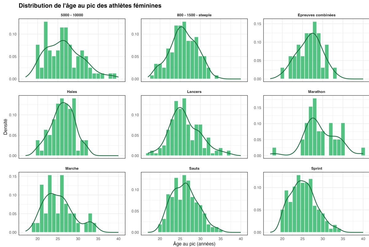
Figure 6: Distributions de l'âge au pic de performance (Athlètes féminines)
