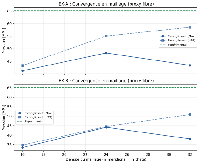
FIGURE 3 – Sensibilité au maillage (Paik EX-A). Le maximum de contrainte strict oscille en raison des singularités géométriques, tandis que le quantile p99 présente une évolution plus stable et monotone.
