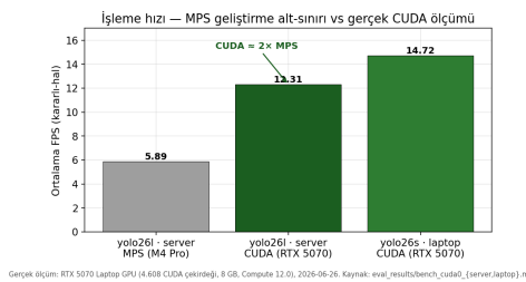
Şekil 6: İşleme hızı: MPS geliştirme alt-sınırı vs gerçek CUDA ölçümü (RTX 5070 Laptop GPU, 4.608 çekirdek, Compute 12.0).
