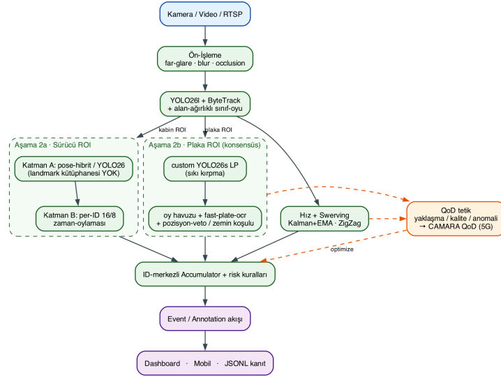
Figure 3: AURA kuşbakışı kaskad boru hattı (kaynak: aura/pipeline/pipeline.py , docs/diagrams/ ).
