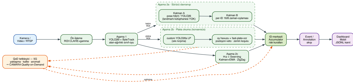
Şekil 3: RoadGuard kuşbakışı kaskad boru hattı (soldan sağa akış): Aşama-1 tespit/takipten iki ROI ile üç paralel Aşama-2 motoruna (sürücü davranışı || plaka okuma || hız) ve ID-merkezli birikime; QoD tetikleyici (kesikli) kritik anda 5G kalitesini talep eder.
