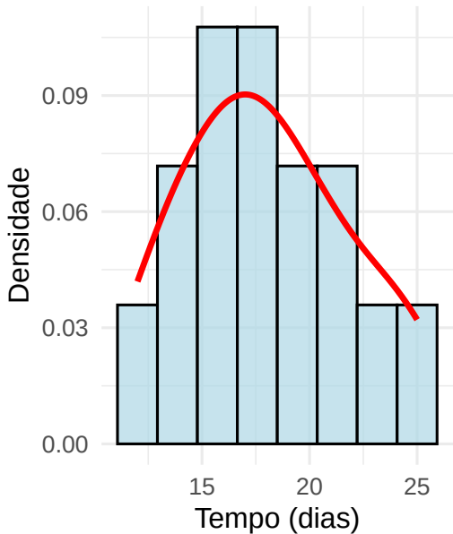
Histograma dos Tempos
