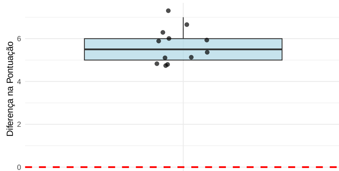
Distribuição das Diferenças
