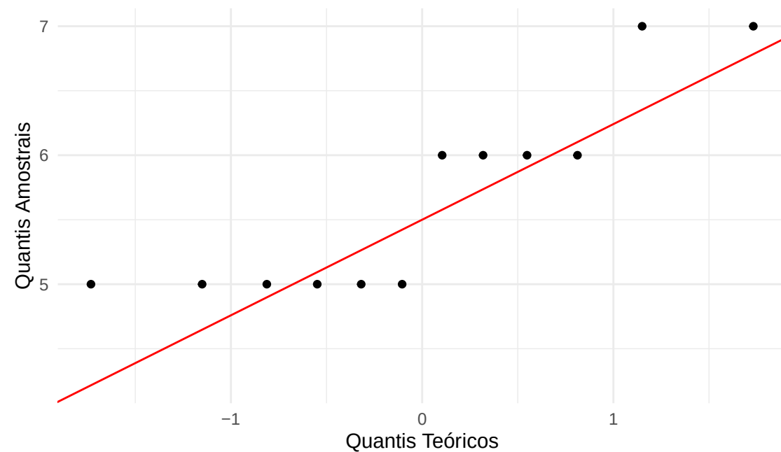
Q-Q Plot das Diferenças
