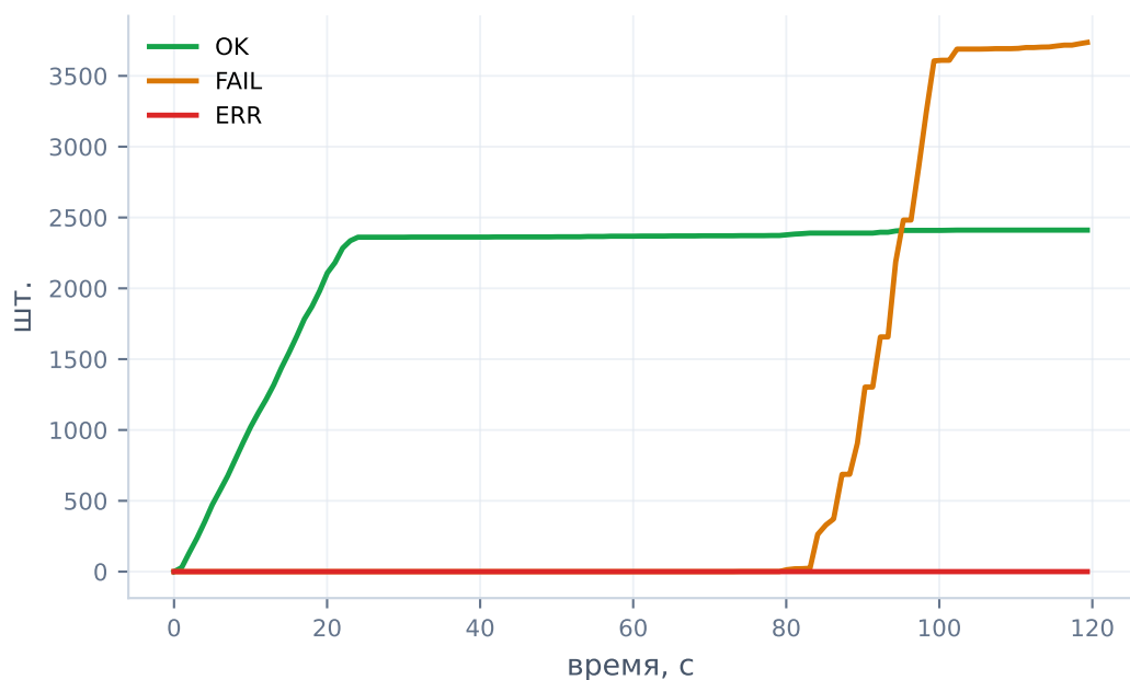
Ответы накопительно
