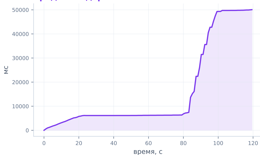
Средняя задержка
