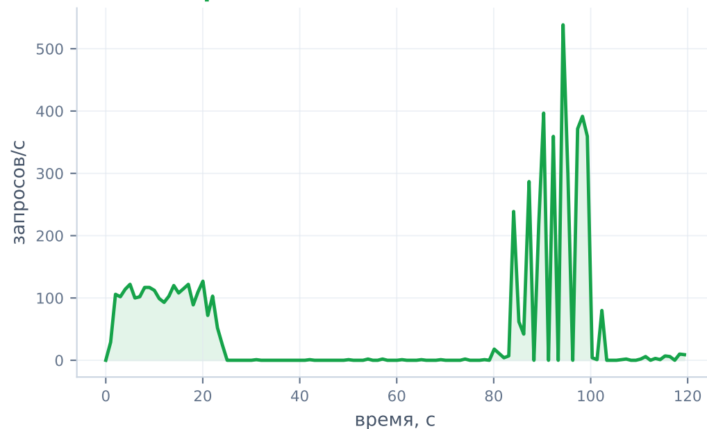
RPS (интервальный)
