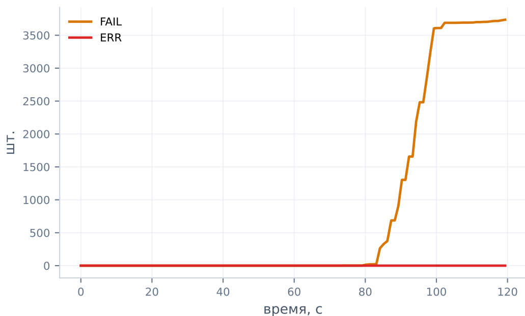
Ошибки накопительно
