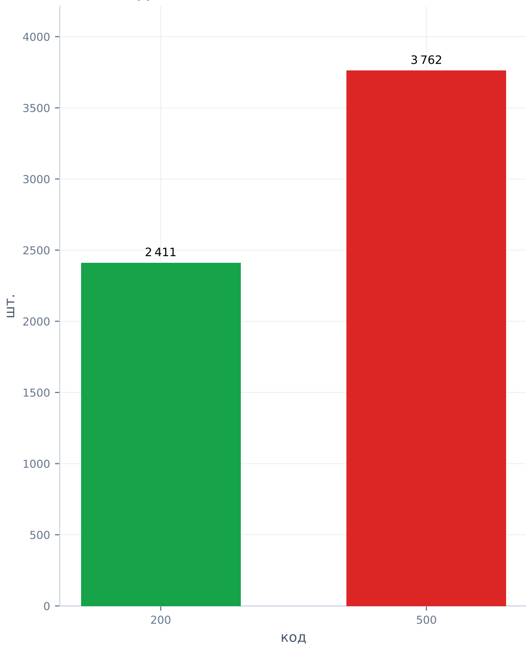
HTTP-коды ответов
