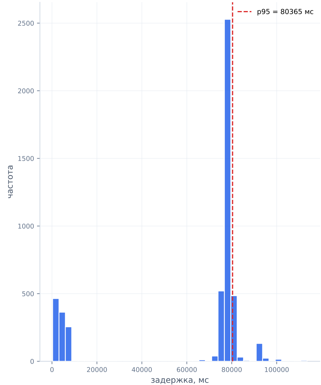
Гистограмма задержек (выборка 4 914)
