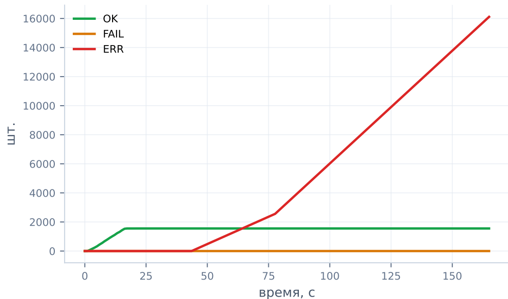
Ответы накопительно
