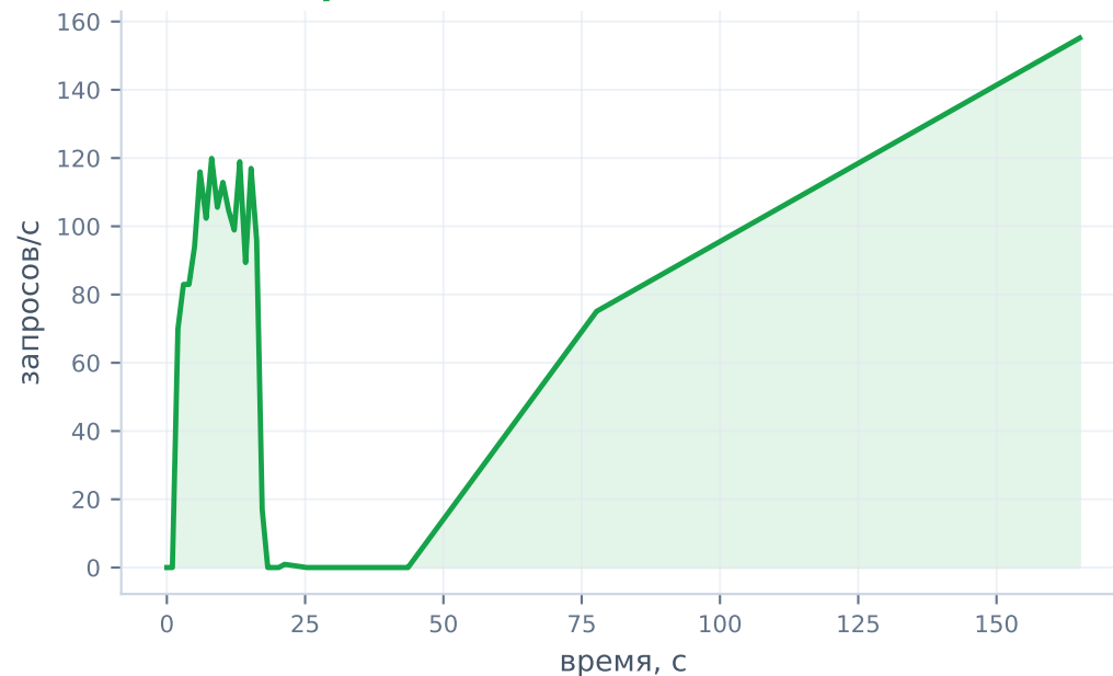
RPS (интервальный)
