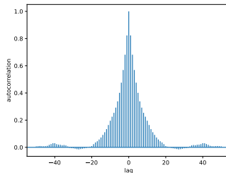
Figure 7: Mauvais autocorrélogramme
