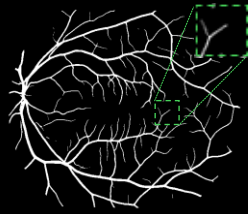
SA-UNetv2
