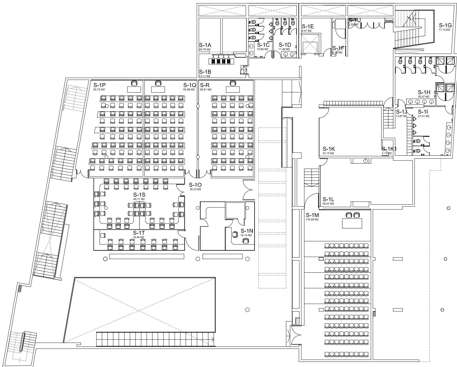
REPUBLICA 180 PLANTA SUBTERRANEO - 1º ESCALA 1:125
