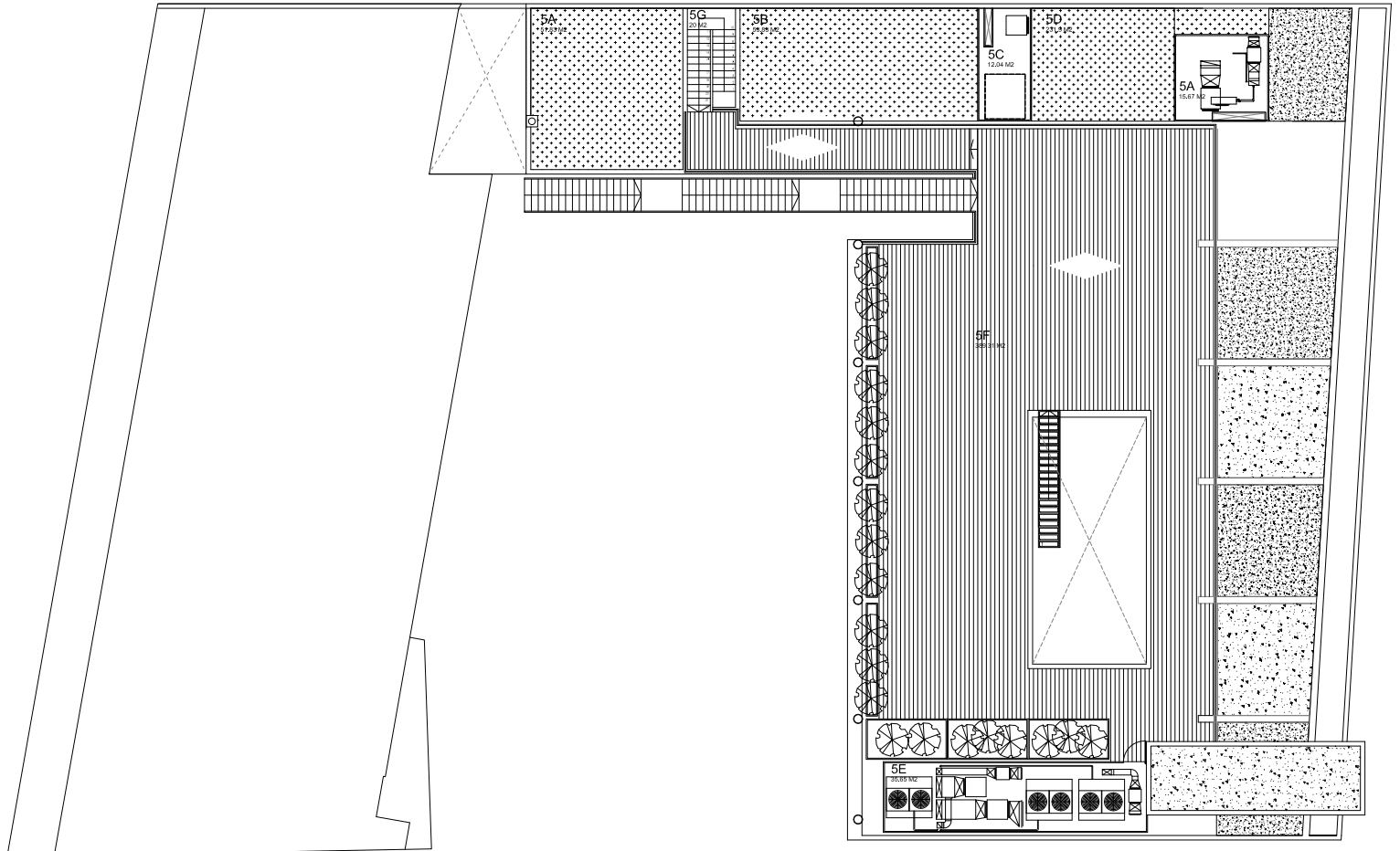
REPUBLICA 180 PLANTA PISO 5 Cubierta ESCALA 1:125
