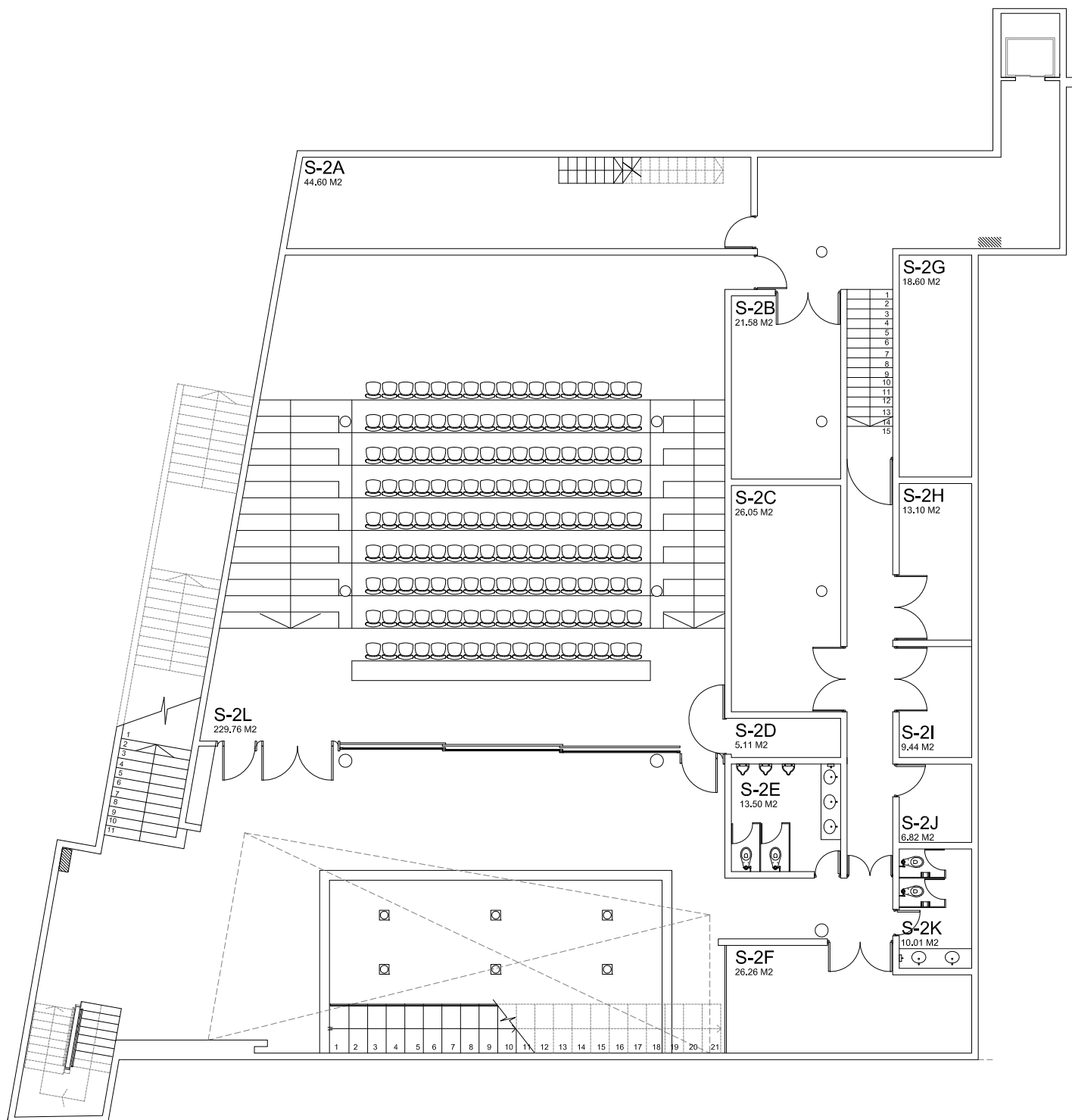
REPUBLICA 180 PLANTA SUBTERRANEO -2° ESCALA 1:125
