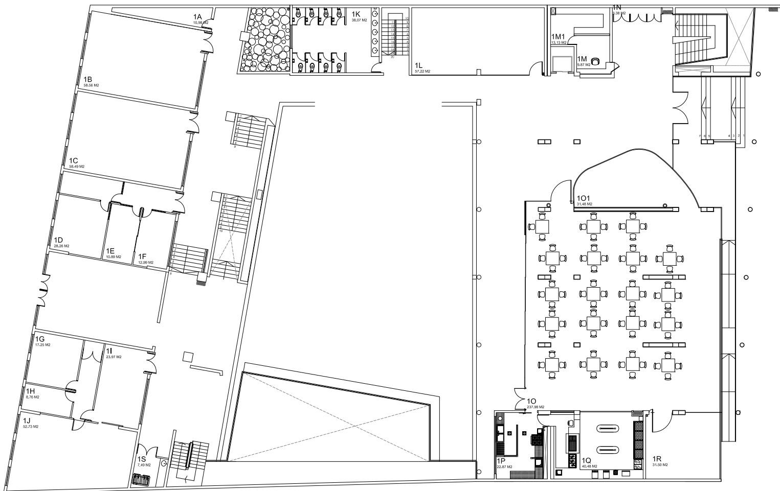
REPUBLICA 180 PLANTA PISO 1 ESCALA 1:125
