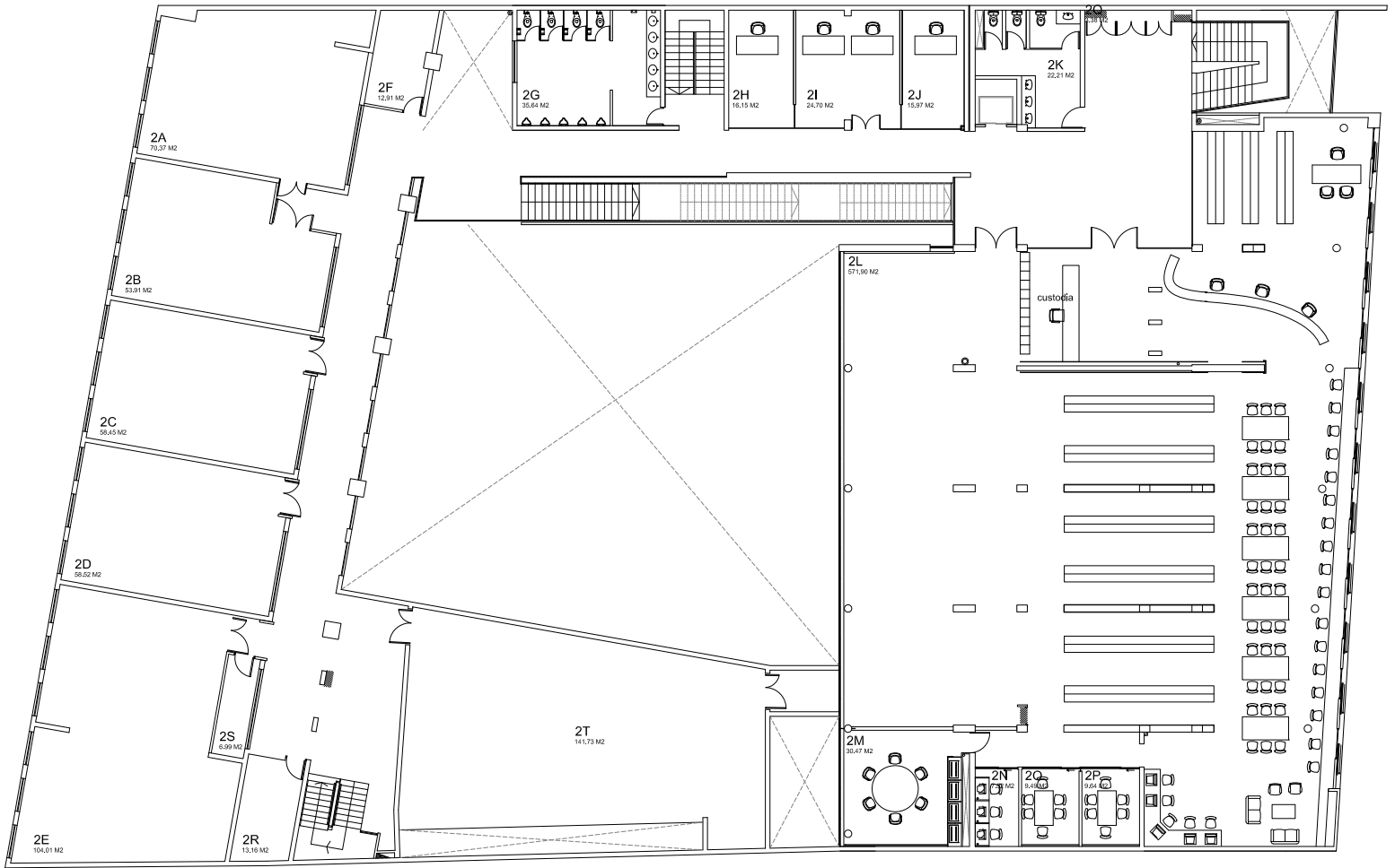
REPUBLICA 180 PLANTA PISO 2 ESCALA 1:125
