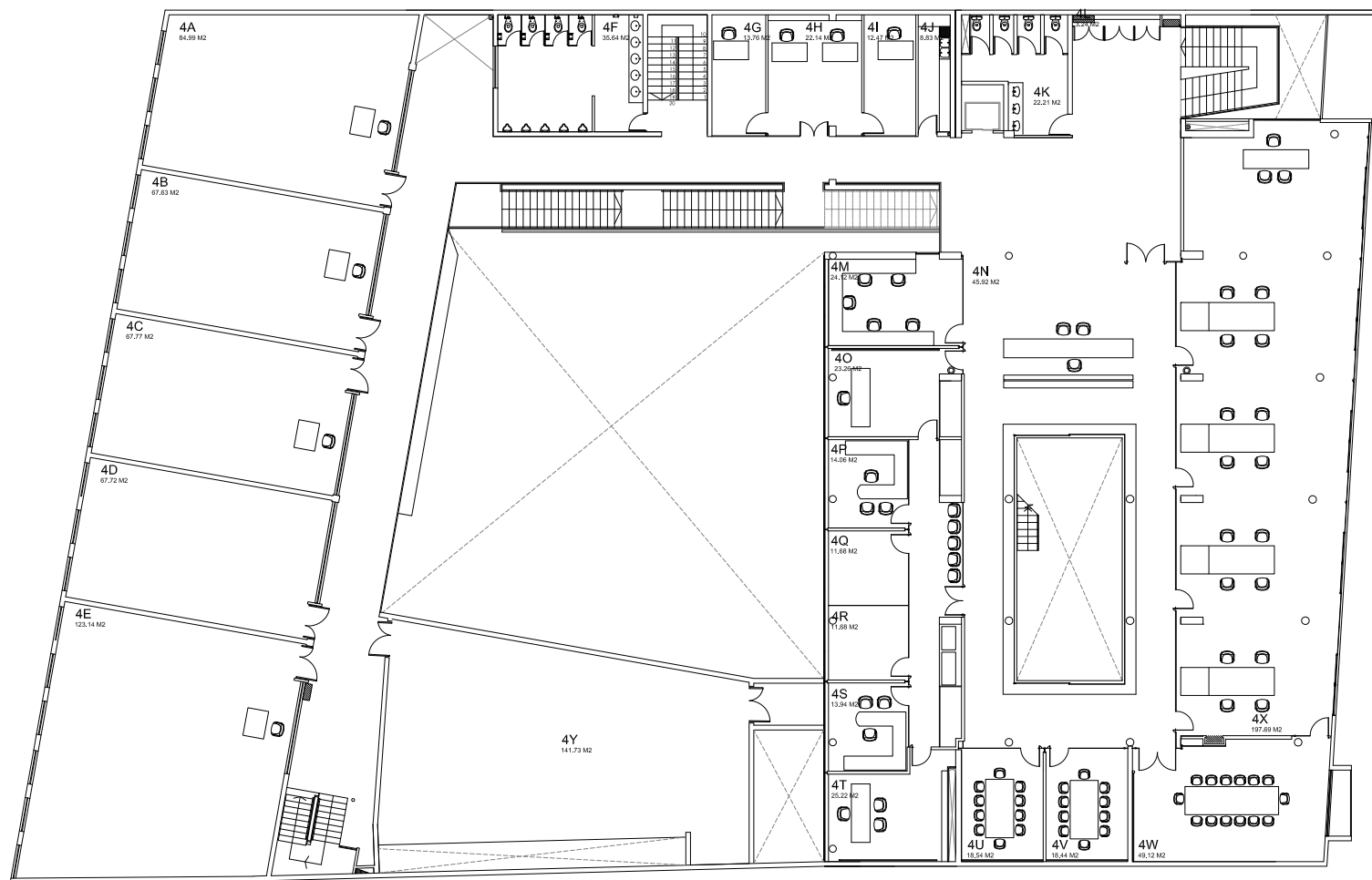
REPUBLICA 180 PLANTA PISO 4 ESCALA 1:125
