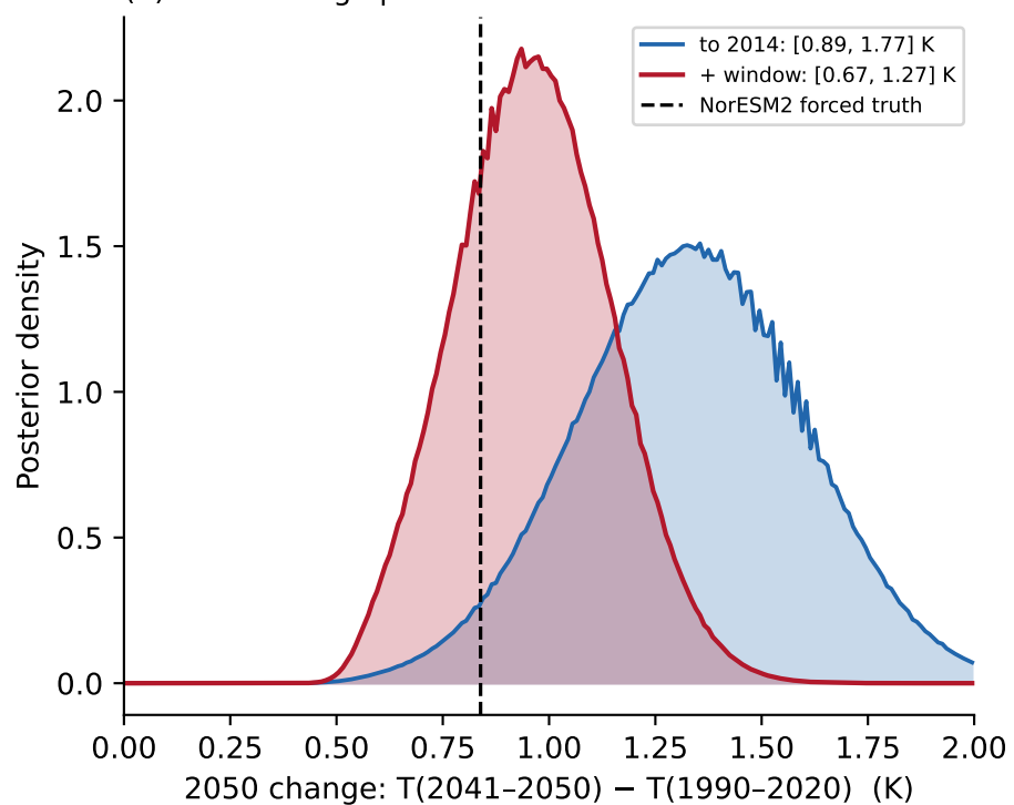
(b) 2050-change posterior
