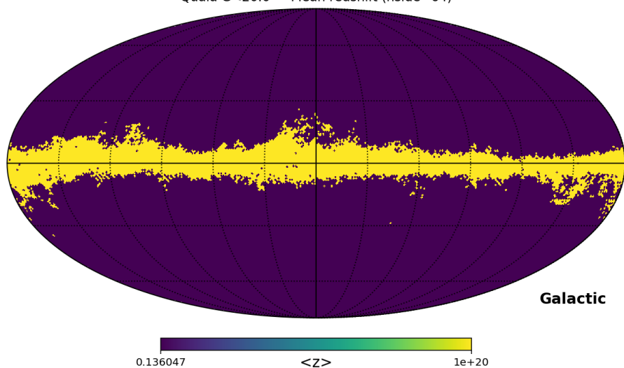
Quiaia G<20.0 — Mean redshift (nside=64)
