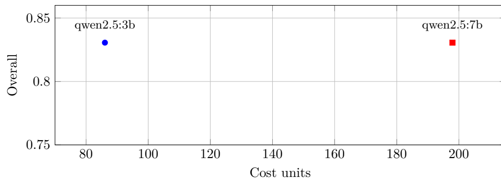
Obr. 3: Graf 2: Pareto cena/kvalita. V tomto behu má 7B rovnaké skóre ako 3B, ale vyšší normalizovaný compute náklad.
