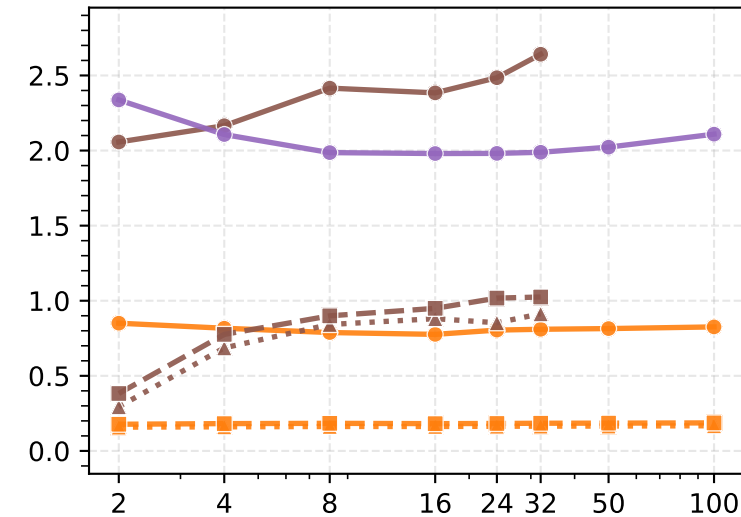
Rays err° ↓
