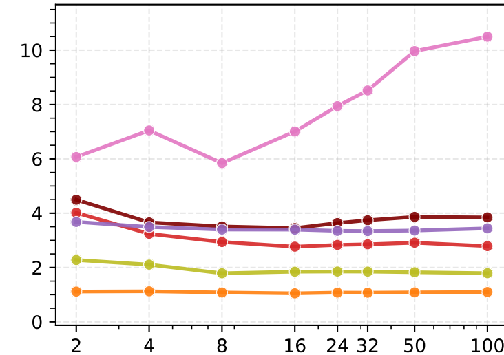
Rays err° ↓
