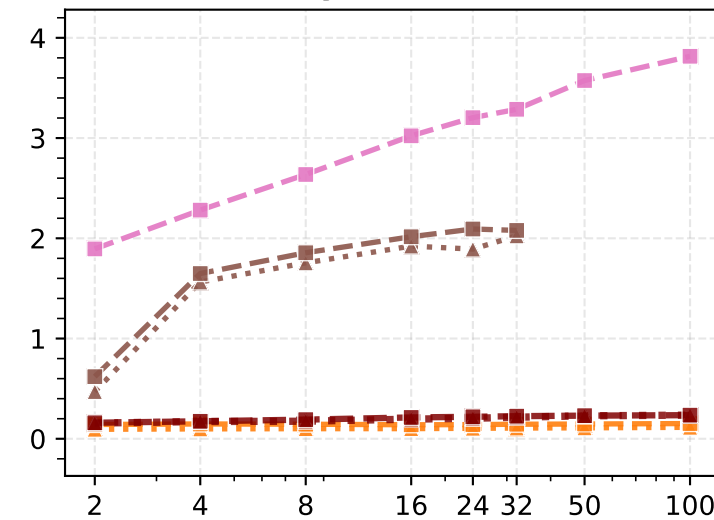
Rays err° ↓
