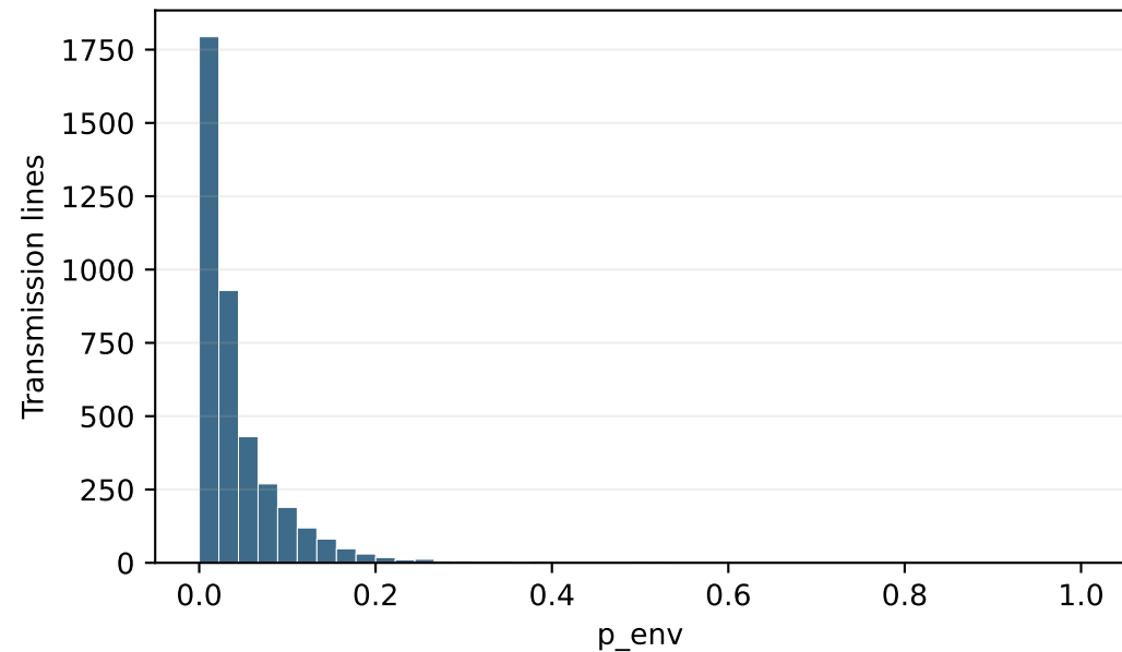
Linear risk
