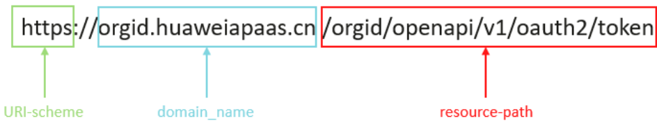
图 3-1 URI 示意图
