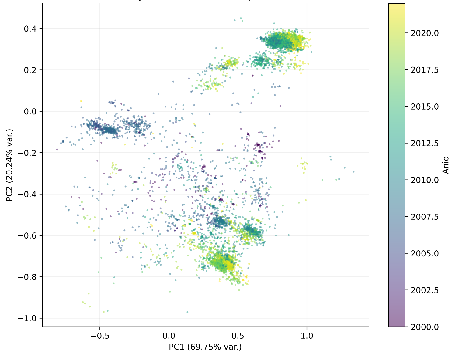
Proyeccion PCA 2D H1N1 por anio
