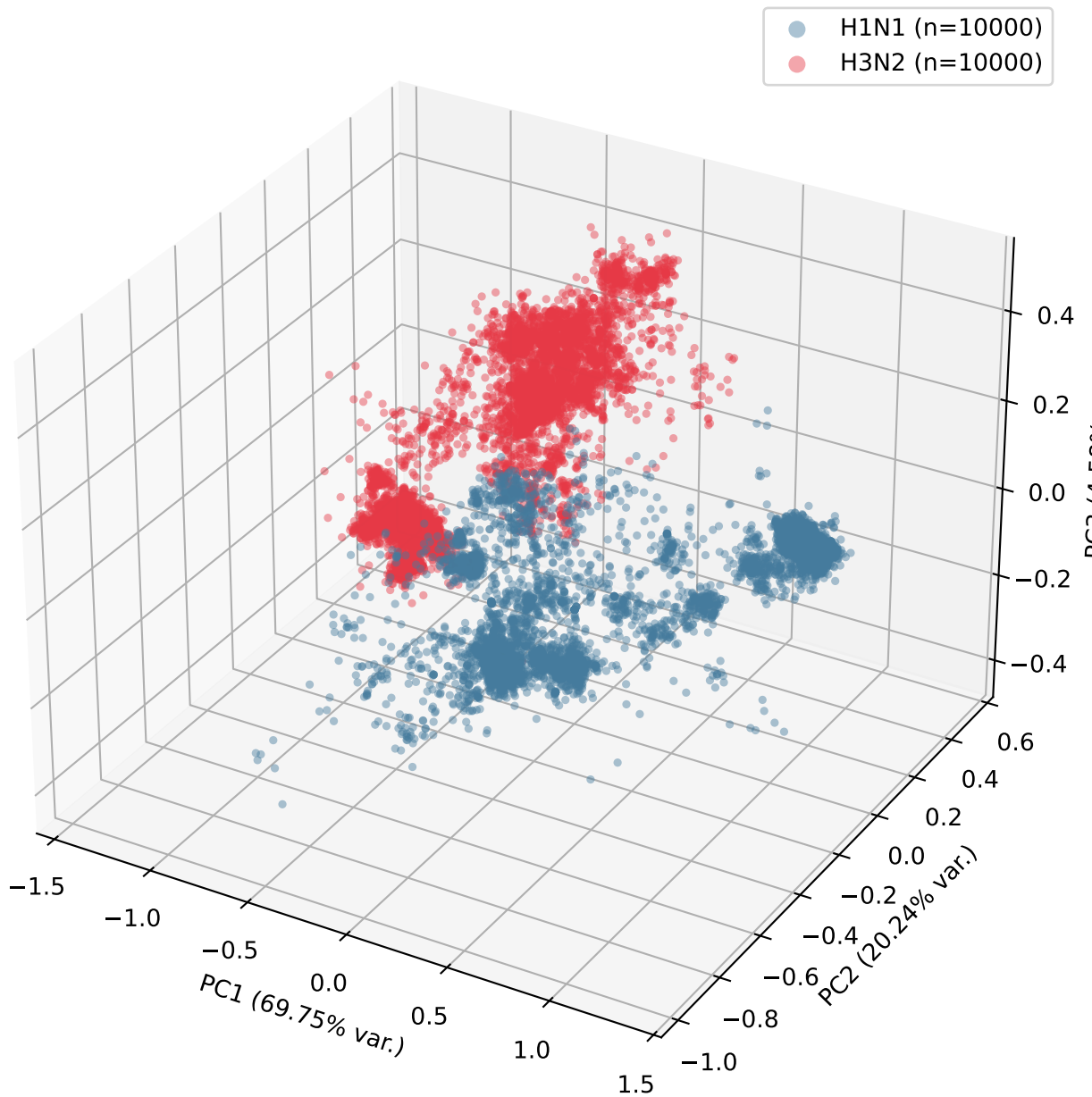
PCA 3D del espacio latente - por subtipo
